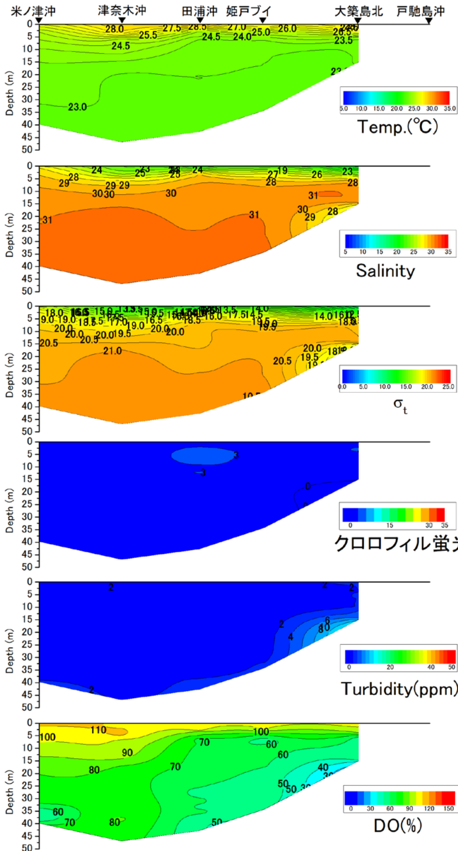
戸馳島沖から米ノ津沖の水温(°C)、塩分、密度( \sigma_t )、クロロフィル蛍光強度、濁度、溶存酸素飽和度(DO%)の鉛直面図(鹿児島県水産技術開発センターの調査による)(2020年8月4日)
