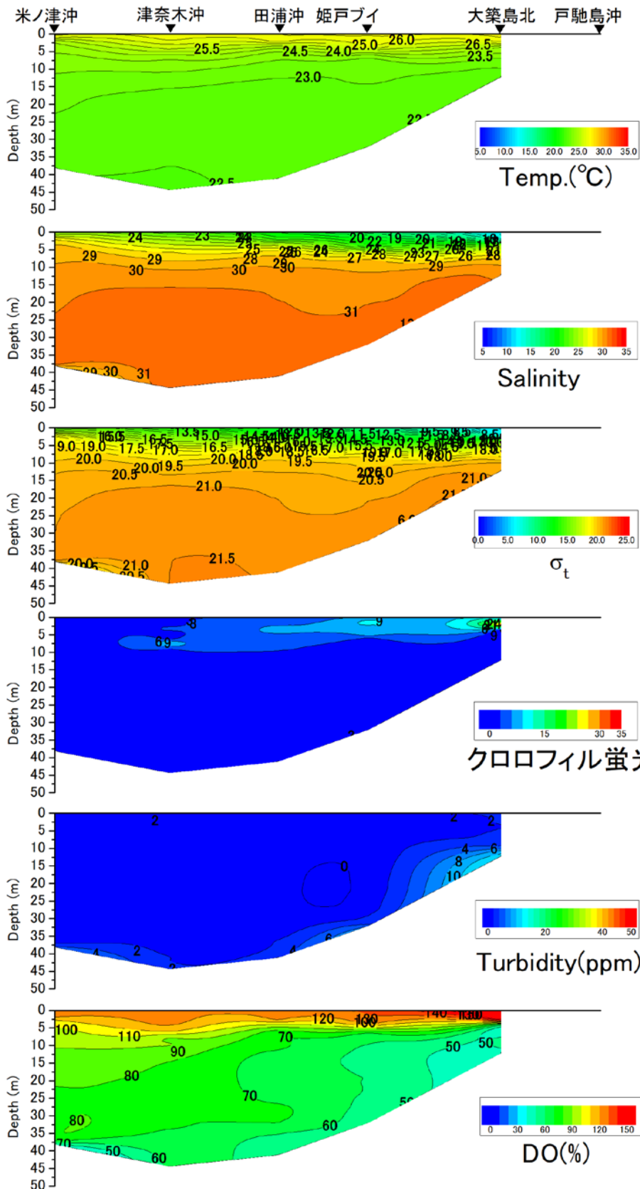
戸馳島沖から米ノ津沖の水温(°C)、塩分、密度( \sigma_t )、クロロフィル蛍光強度、濁度、溶存酸素飽和度(DO%)の鉛直面図(鹿児島県水産技術開発センターの調査による)(2020年7月29日)
