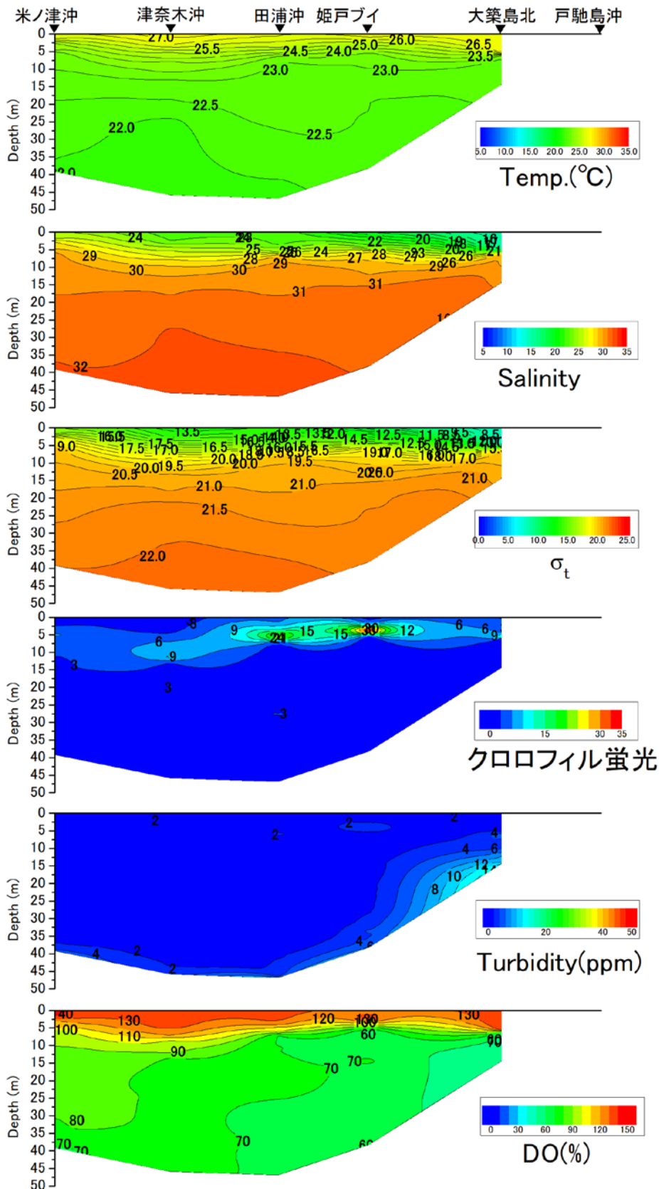
戸馳島沖から米ノ津沖の水温 (°C)、塩分、密度 ( \sigma_t )、クロロフィル蛍光強度、濁度、溶存酸素飽和度 (DO%) の鉛直面図 (熊本県水産研究センターの調査による) (2020年7月21日)
