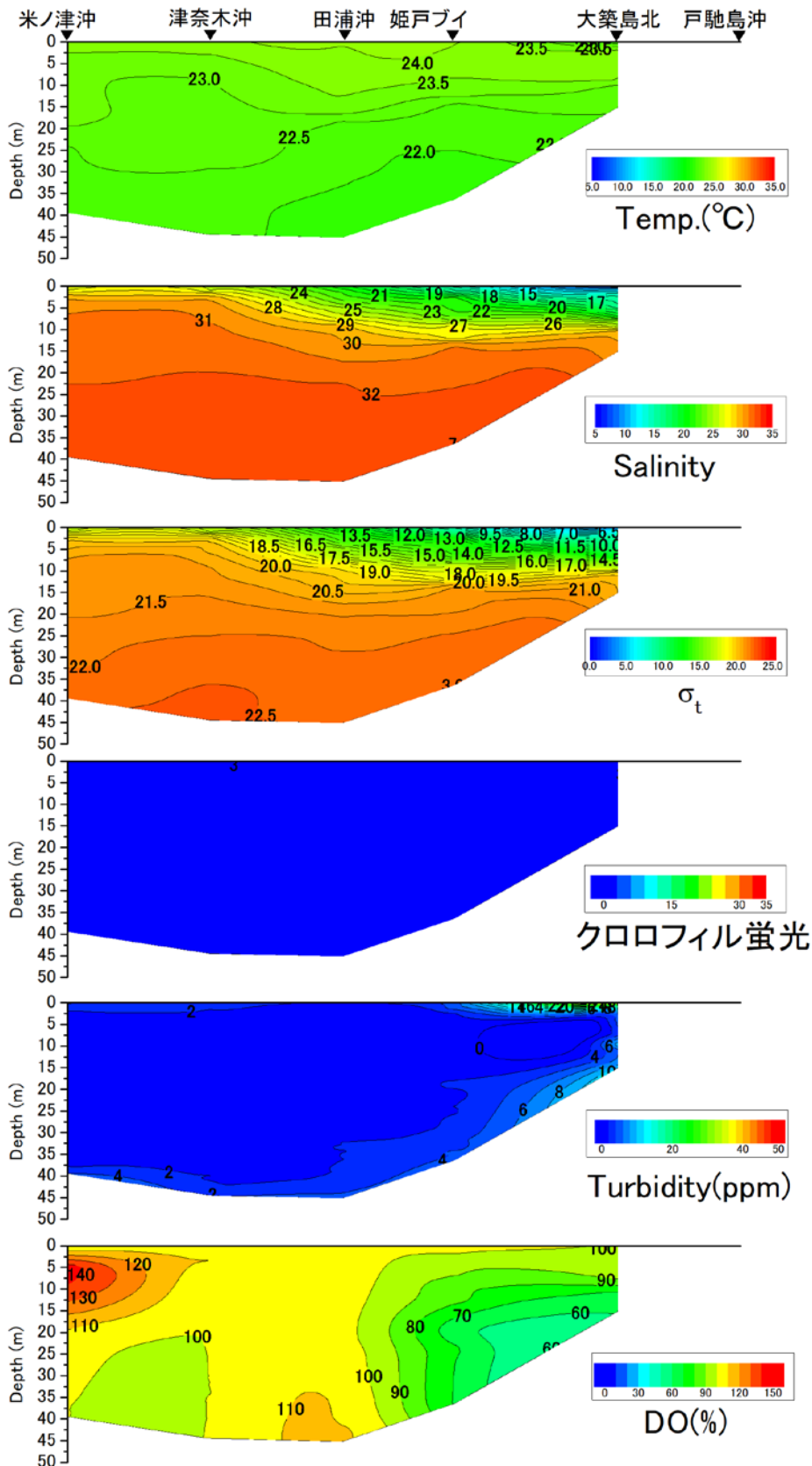
戸馳島沖から米ノ津沖の水温 (°C)、塩分、密度 ( \sigma_t )、クロロフィル蛍光強度、濁度、溶存酸素飽和度 (DO%) の鉛直面図 (東町漁業協同組合の調査による) (2020年7月8日)
