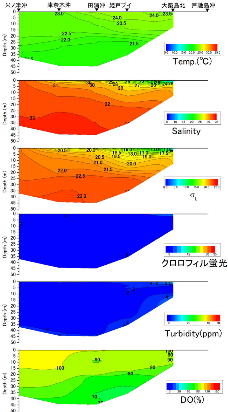
戸馳島沖から米ノ津沖の水温 (°C)、塩分、密度 ( \sigma_t )、クロロフィル蛍光強度、濁度、溶存酸素飽和度 (DO%) の鉛直面図 (熊本県水産研究センターの調査による) (2020年7月1日)
