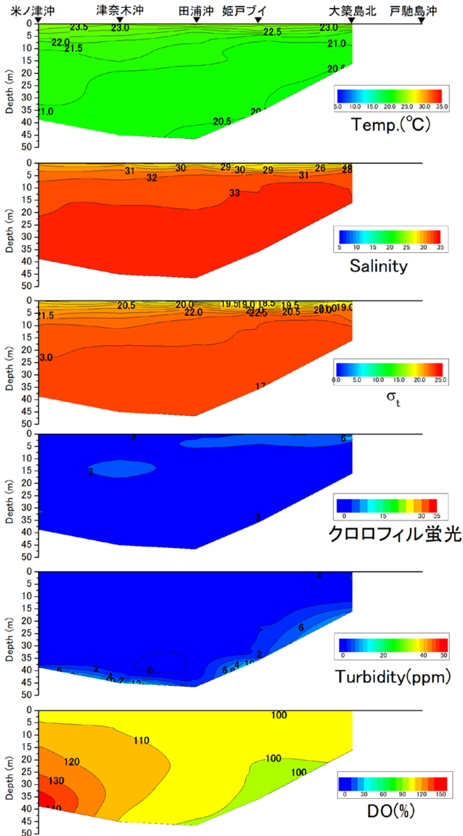
戸馳島沖から米ノ津沖の水温 (°C)、塩分、密度 ( \sigma_t )、クロロフィル蛍光強度、濁度、溶存酸素飽和度 (DO%) の鉛直面図 (東町漁業協同組合の調査による) (2020年6月23日)
