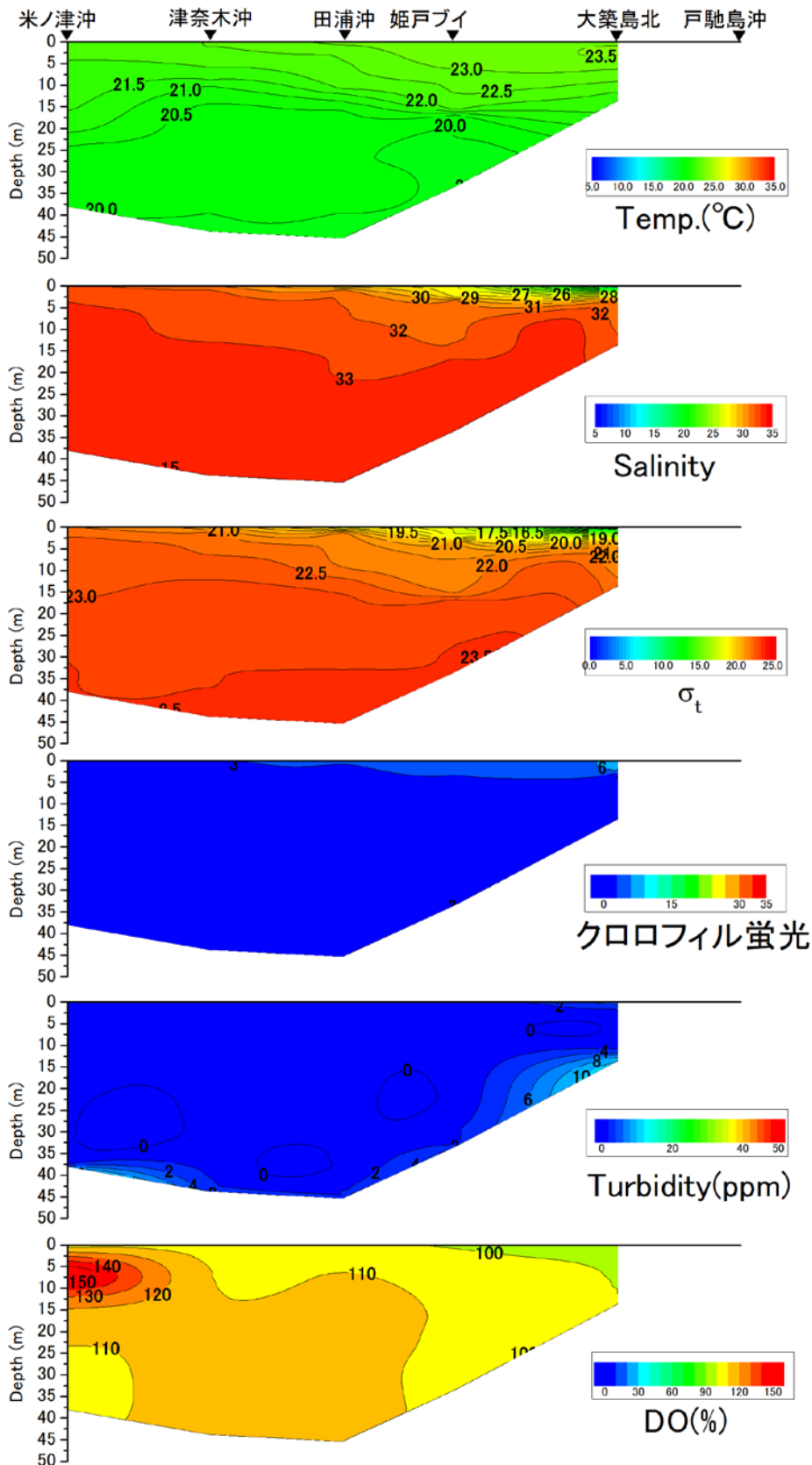
戸馳島沖から米ノ津沖の水温 (°C)、塩分、密度 ( \sigma_t )、クロロフィル蛍光強度、濁度、溶存酸素飽和度 (DO%) の鉛直面図 (東町漁業協同組合の調査による) (2020年6月16日)
