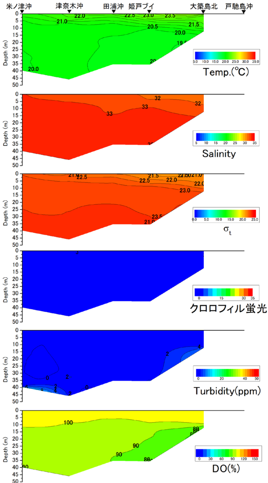
戸馳島沖から米ノ津沖の水温 (°C)、塩分、密度 ( \sigma_t )、クロロフィル蛍光強度、濁度、溶存酸素飽和度 (DO%) の鉛直面図 (熊本県水産研究センターの調査による) (2020年6月9日)
