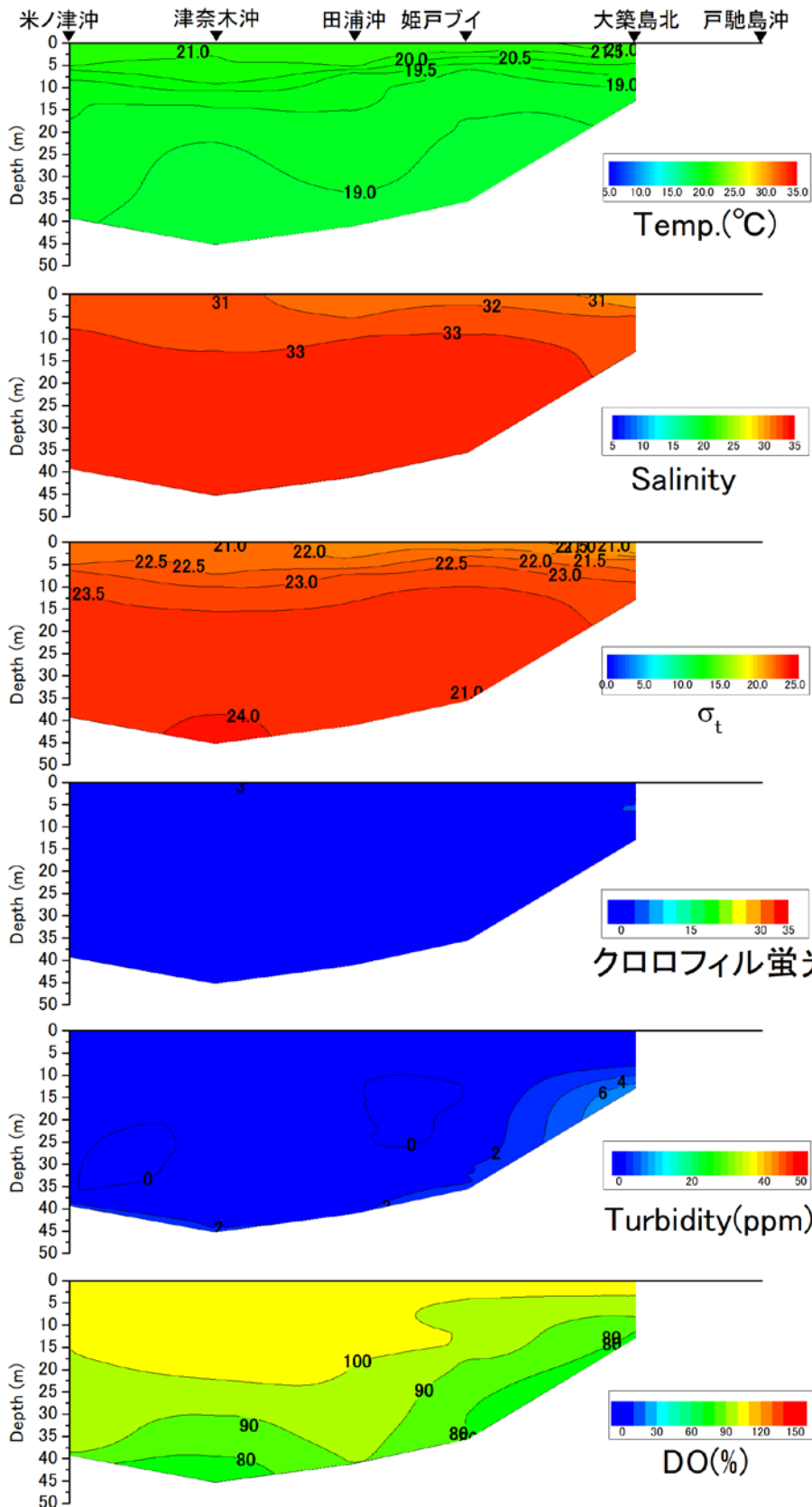
戸馳島沖から米ノ津沖の水温(°C)、塩分、密度( \sigma_t )、クロロフィル蛍光強度、濁度、溶存酸素飽和度(DO%)の鉛直面図(鹿児島県水産技術開発センターの調査による)(2020年6月2日)
