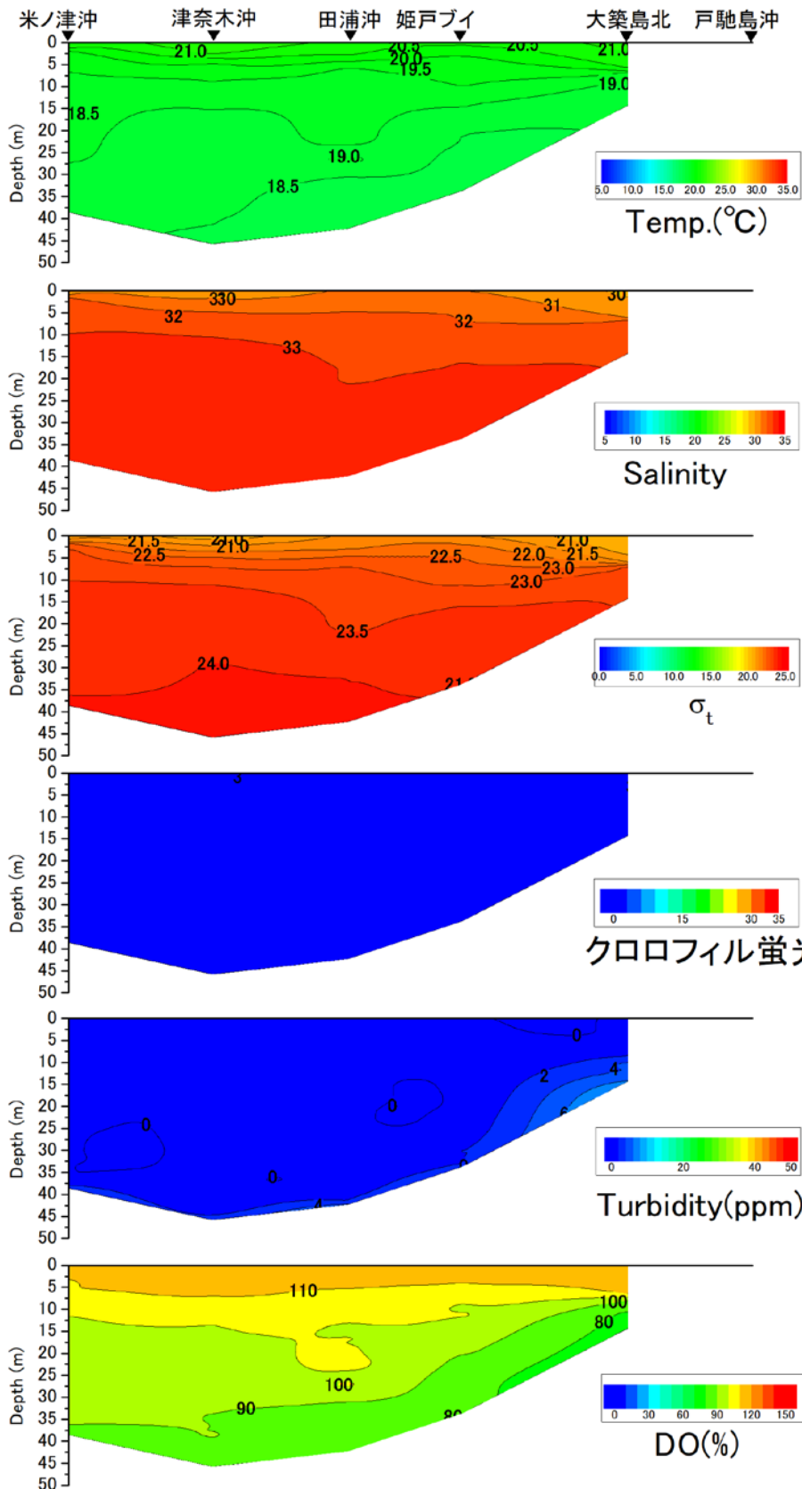
戸馳島沖から米ノ津沖の水温(°C)、塩分、密度( \sigma_t )、クロロフィル蛍光強度、濁度、溶存酸素飽和度(DO%)の鉛直面図(鹿児島県水産技術開発センターの調査による)(2020年5月27日)
