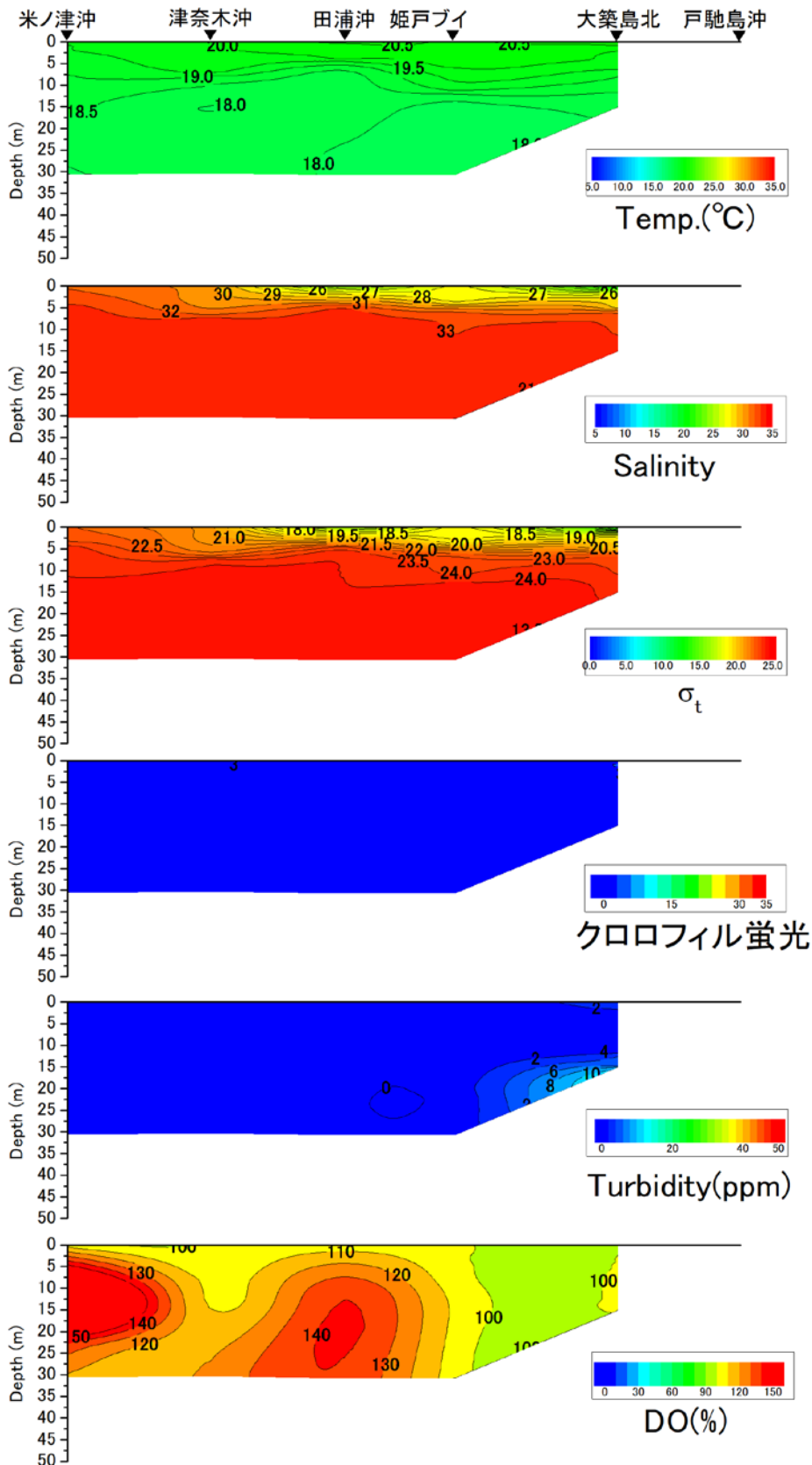
戸馳島沖から米ノ津沖の水温 (°C)、塩分、密度 ( \sigma_t )、クロロフィル蛍光強度、濁度、溶存酸素飽和度 (DO%) の鉛直面図 (東町漁業協同組合の調査による) (2020年5月19日)
