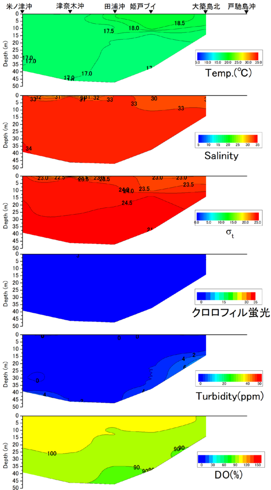
戸馳島沖から米ノ津沖の水温 (°C)、塩分、密度 ( \sigma_t )、クロロフィル蛍光強度、濁度、溶存酸素飽和度 (DO%) の鉛直面図 (熊本県水産研究センターの調査による) (2020年5月7日)
