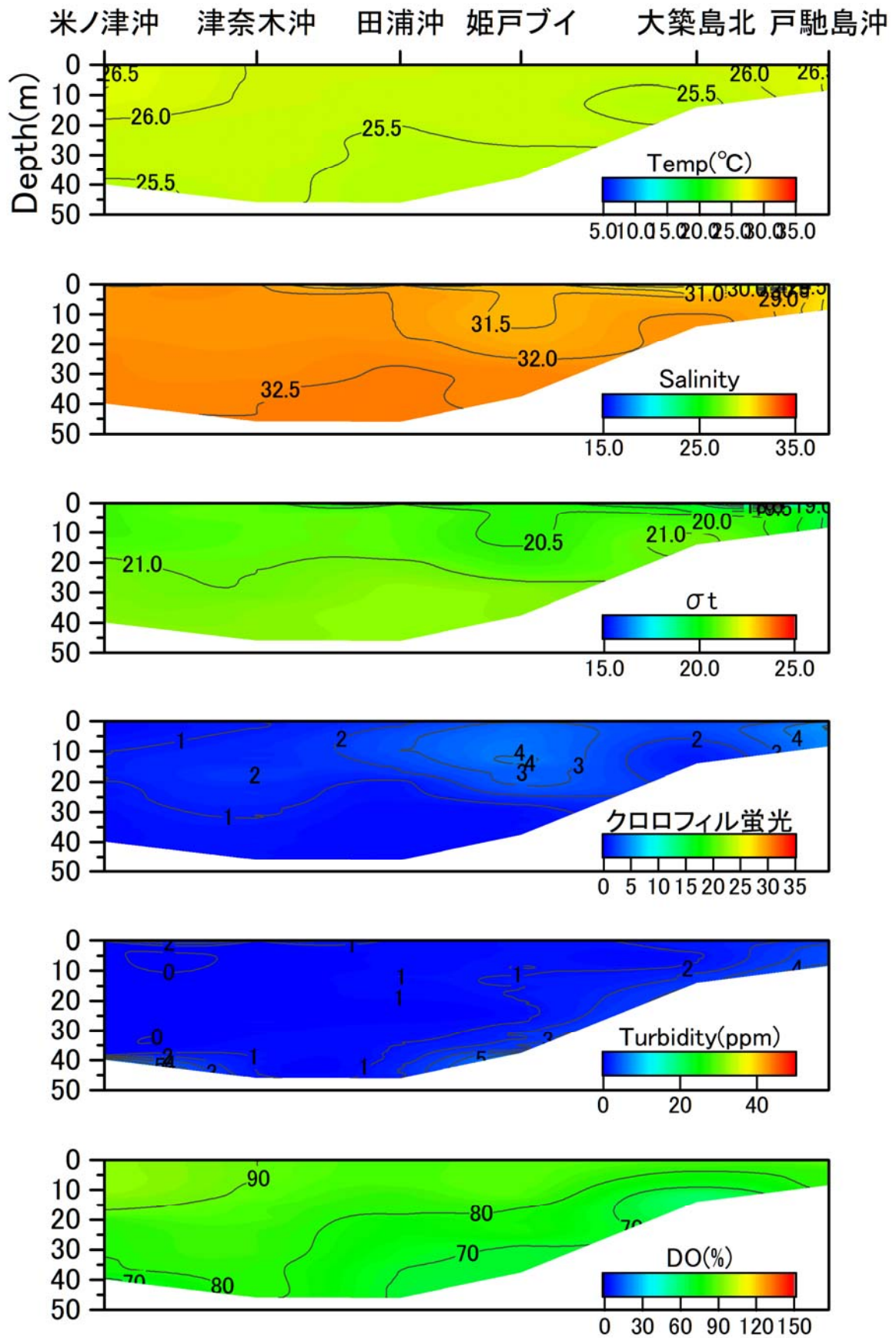
戸馳島沖から米ノ津沖の水温 (°C)、塩分、密度 ( \sigma_t )、クロロフィル蛍光強度、濁度、溶存酸素飽和度 (DO%) の鉛直面図 (熊本県水産研究センターの調査による) (2019年9月17日)
