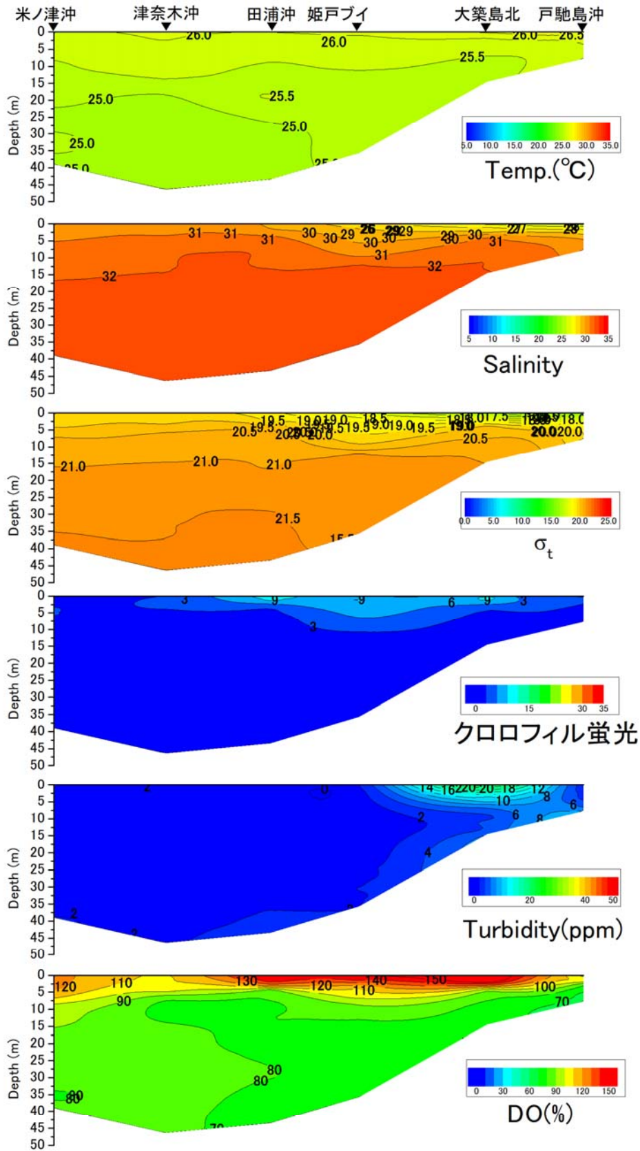
戸馳島沖から米ノ津沖の水温(°C)、塩分、密度( \sigma_t )、クロロフィル蛍光強度、濁度、溶存酸素飽和度(DO%)の鉛直面図(鹿児島県水産技術開発センターの調査による)(2019年9月3日)
