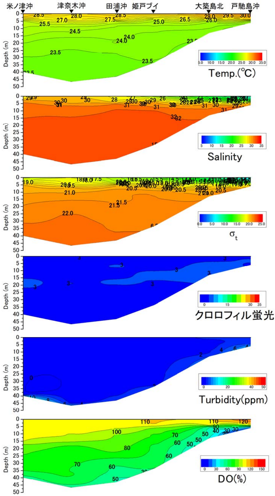
戸馳島沖から米ノ津沖の水温(°C)、塩分、密度( \sigma_t )、クロロフィル蛍光強度、濁度、溶存酸素飽和度(DO%)の鉛直面図(鹿児島県水産技術開発センターの調査による)(2019年7月30日)
