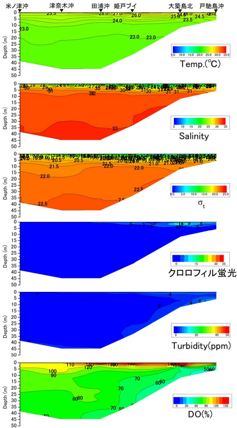
戸馳島沖から米ノ津沖の水温 (°C)、塩分、密度 ( \sigma_t )、クロロフィル蛍光強度、濁度、溶存酸素飽和度 (DO%) の鉛直面図 (熊本県水産研究センターの調査による) (2019年7月16日)
