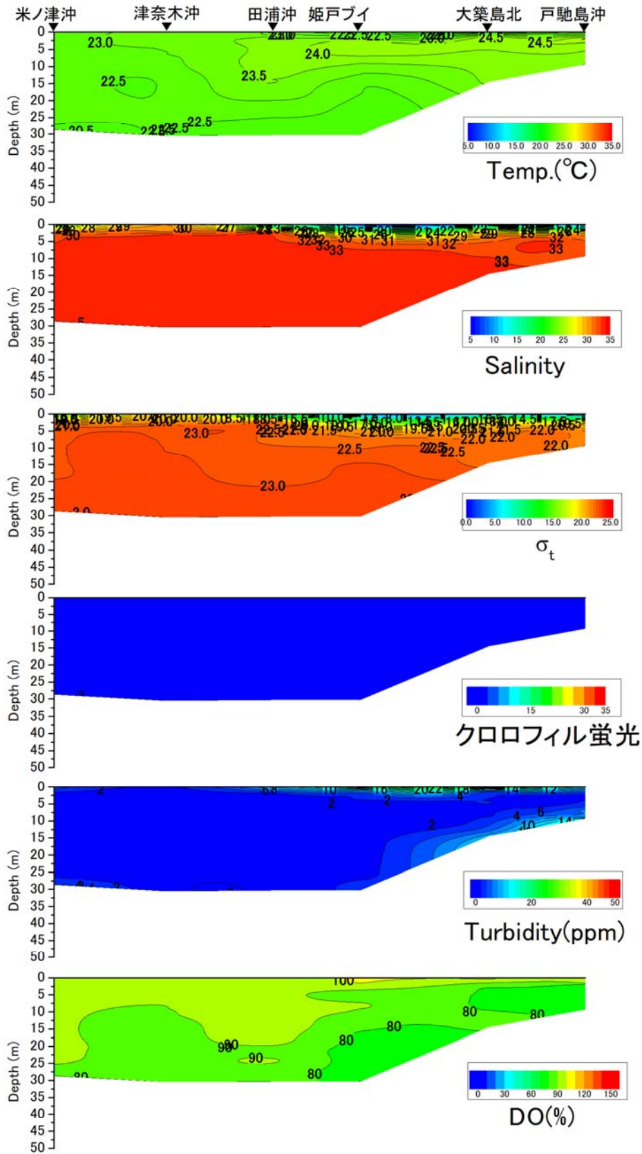
戸馳島沖から米ノ津沖の水温 (°C) 、塩分、密度 ( \sigma_t ) 、クロロフィル 蛍光強度、濁度、溶存酸素飽和度 (DO%) の鉛直面図 (東町漁業協同組 合の調査による) (2019年7月2日)
