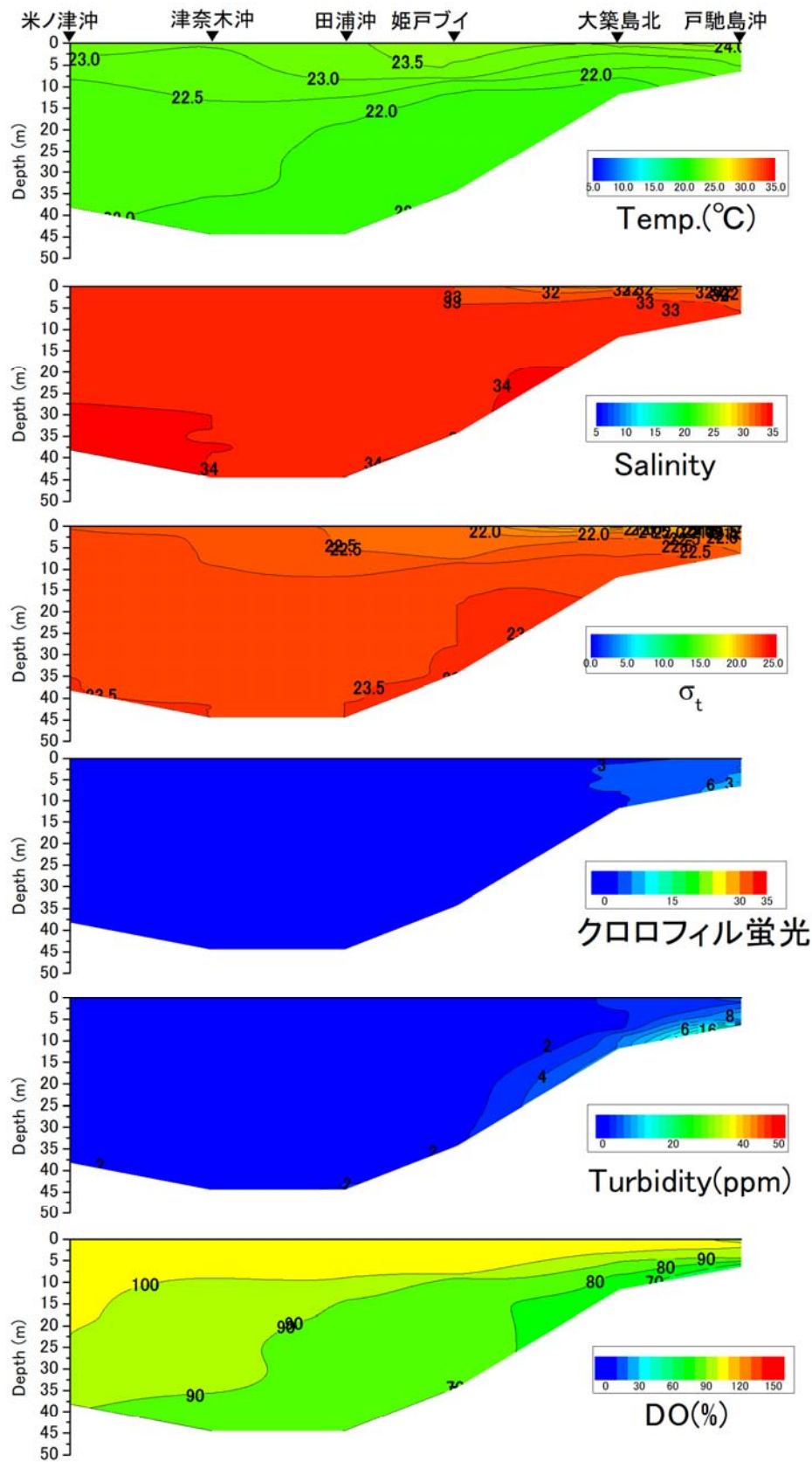
戸馳島沖から米ノ津沖の水温 (°C)、塩分、密度 ( \sigma_t )、クロロフィル蛍光強度、濁度、溶存酸素飽和度 (DO%) の鉛直面図 (熊本県水産研究センターの調査による) (2019年6月25日)
