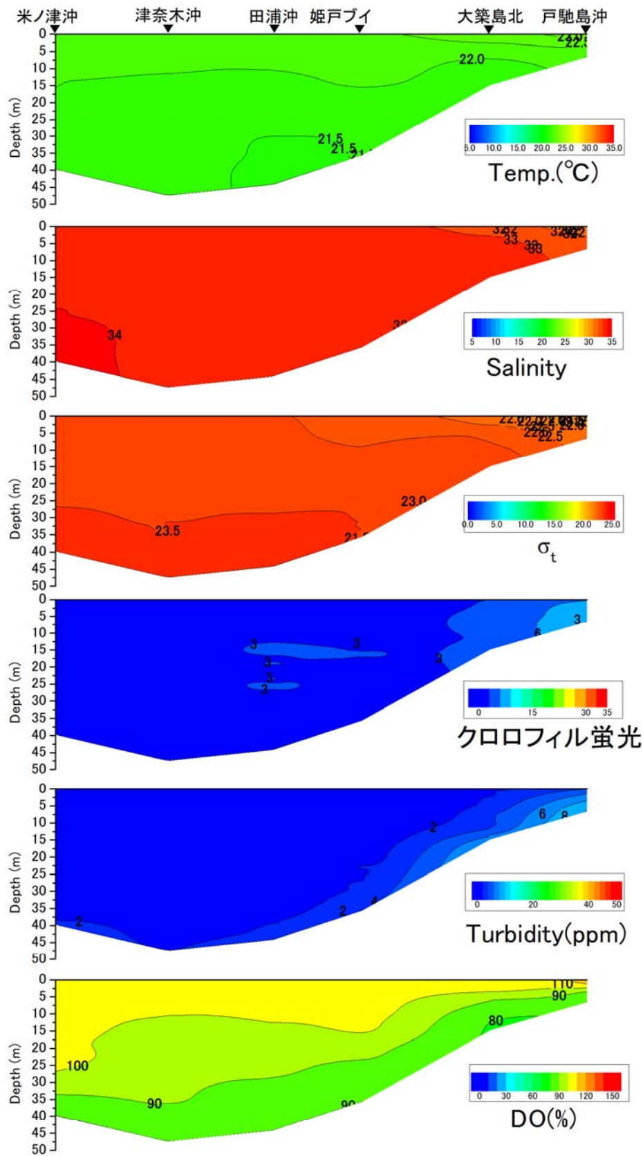
戸馳島沖から米ノ津沖の水温(°C)、塩分、密度( \sigma_t )、クロロフィル蛍光強度、濁度、溶存酸素飽和度(DO%)の鉛直面図(鹿児島県水産技術開発センターの調査による)(2019年6月18日)
