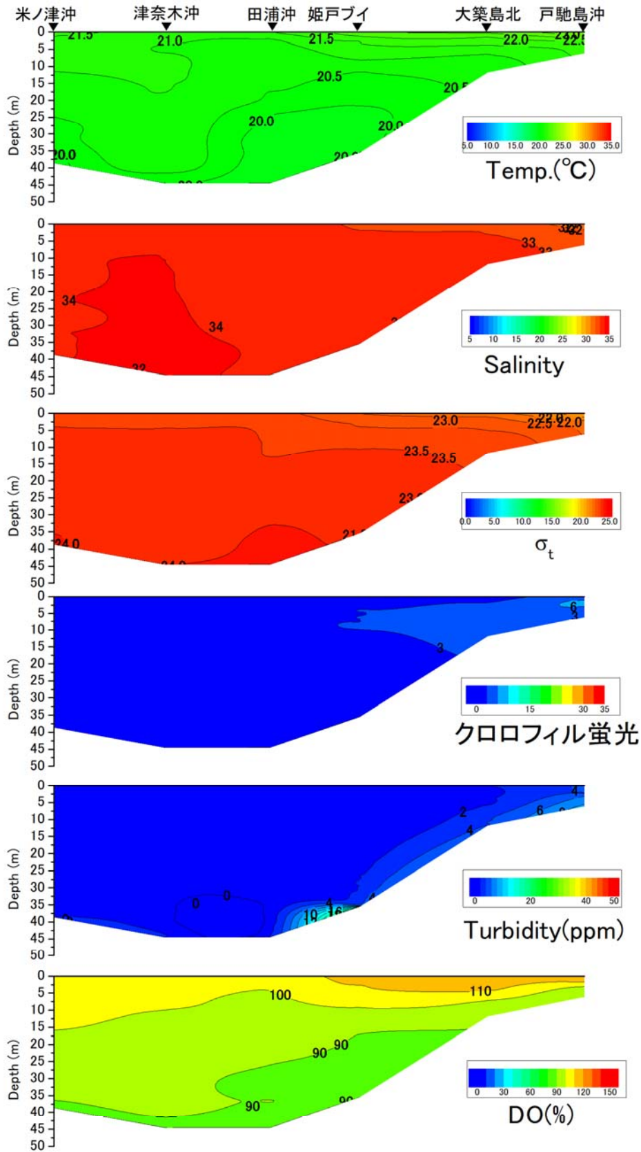
戸馳島沖から米ノ津沖の水温 (°C)、塩分、密度 ( \sigma_t )、クロロフィル蛍光強度、濁度、溶存酸素飽和度 (DO%) の鉛直面図 (熊本県水産研究センターの調査による) (2019年6月4日)
