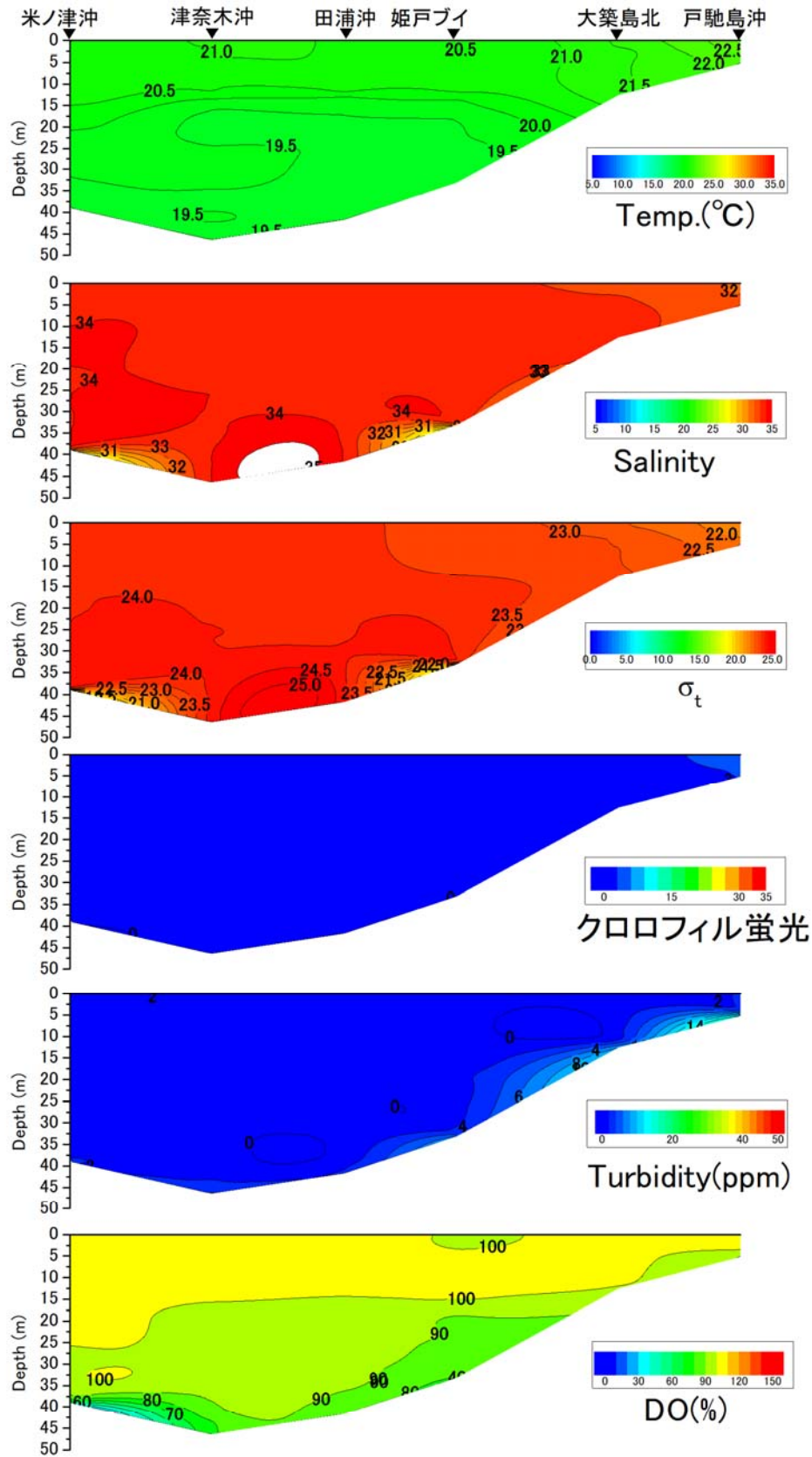
戸馳島沖から米ノ津沖の水温(°C)、塩分、密度( \sigma_t )、クロロフィル蛍光強度、濁度、溶存酸素飽和度(DO%)の鉛直面図(鹿児島県水産技術開発センターの調査による)(2019年5月28日)
