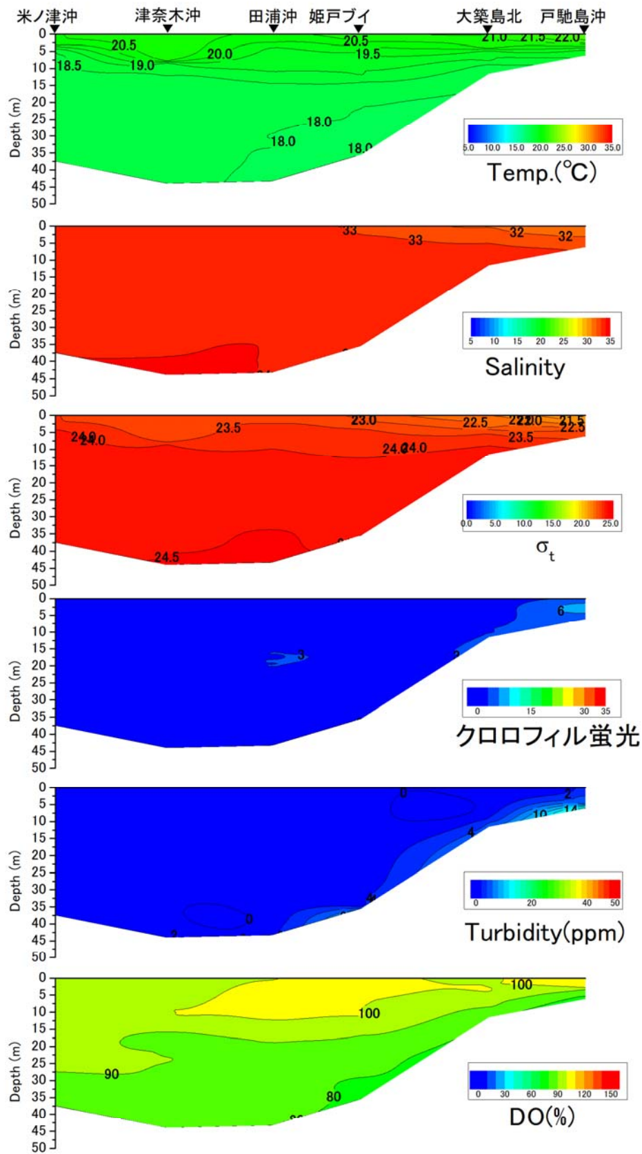
戸馳島沖から米ノ津沖の水温 (°C)、塩分、密度 ( \sigma_t )、クロロフィル蛍光強度、濁度、溶存酸素飽和度 (DO%) の鉛直面図 (熊本県水産研究センターの調査による) (2019年5月14日)
