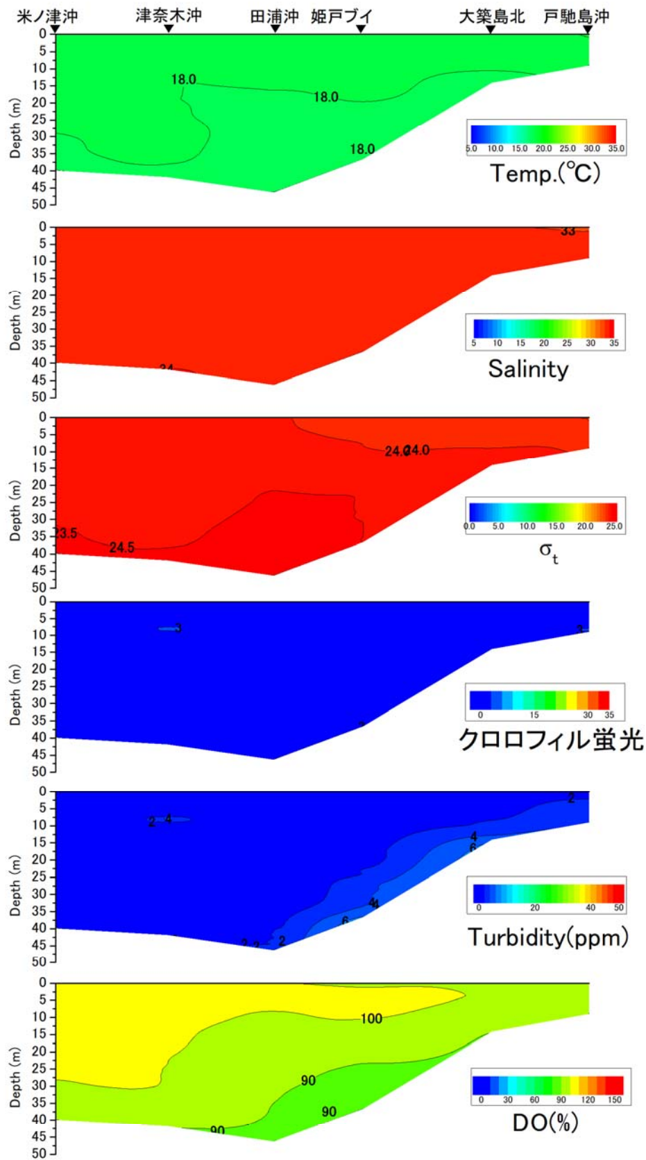
戸馳島沖から米ノ津沖の水温(°C)、塩分、密度( \sigma_t )、クロロフィル蛍光強度、濁度、溶存酸素飽和度(DO%)の鉛直面図(鹿児島県水産技術開発センターの調査による)(2019年5月8日)
