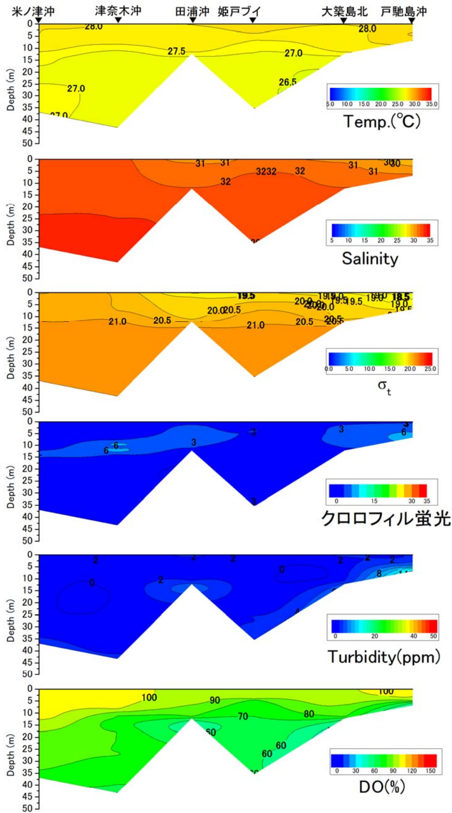
戸馳島沖から米ノ津沖の水温(°C)、塩分、密度( \sigma_t )、クロロフィル蛍光強度、濁度、溶存酸素飽和度(DO%)の鉛直面図(熊本県水産研究センターの調査による)(2018年9月6日)
