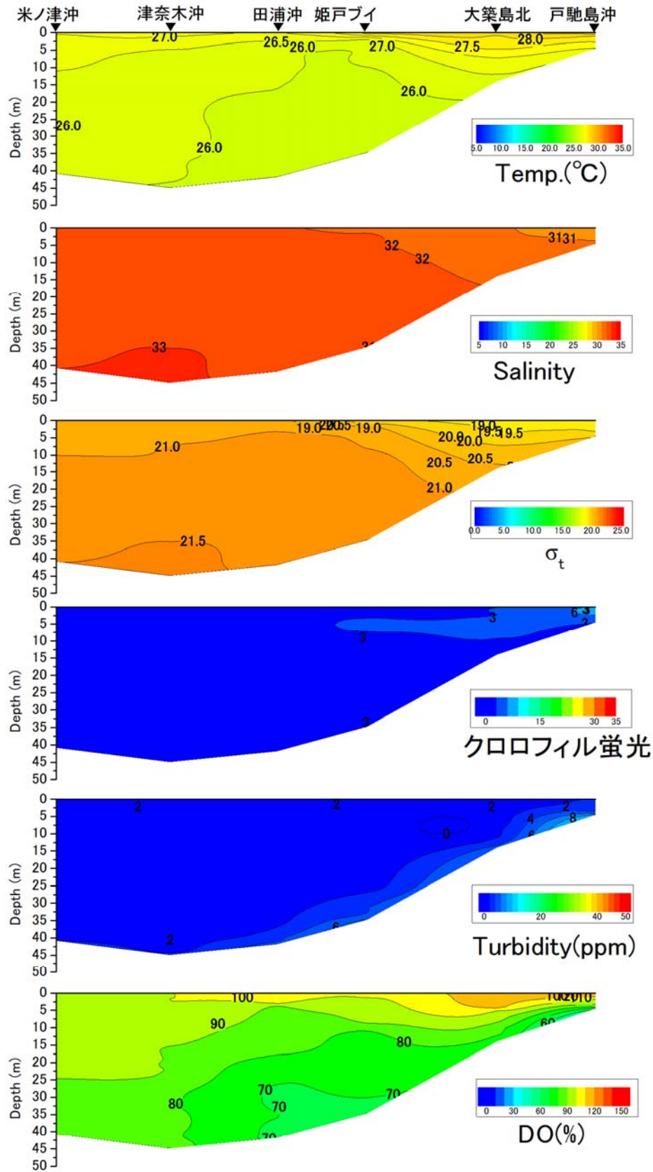
戸馳島沖から米ノ津沖の水温(°C)、塩分、密度( \sigma_t )、クロロフィル蛍光強度、濁度、溶存酸素飽和度(DO%)の鉛直面図(鹿児島県水産技術開発センターの調査による)(2018年8月23日)
