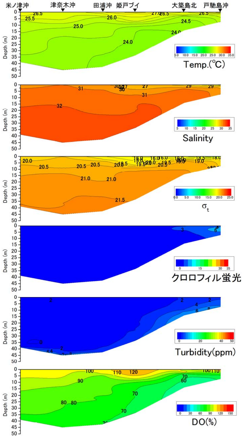
戸馳島沖から米ノ津沖の水温(°C)、塩分、密度( \sigma_t )、クロロフィル蛍光強度、濁度、溶存酸素飽和度(DO%)の鉛直面図(鹿児島県水産技術開発センターの調査による)(2018年8月2日)
