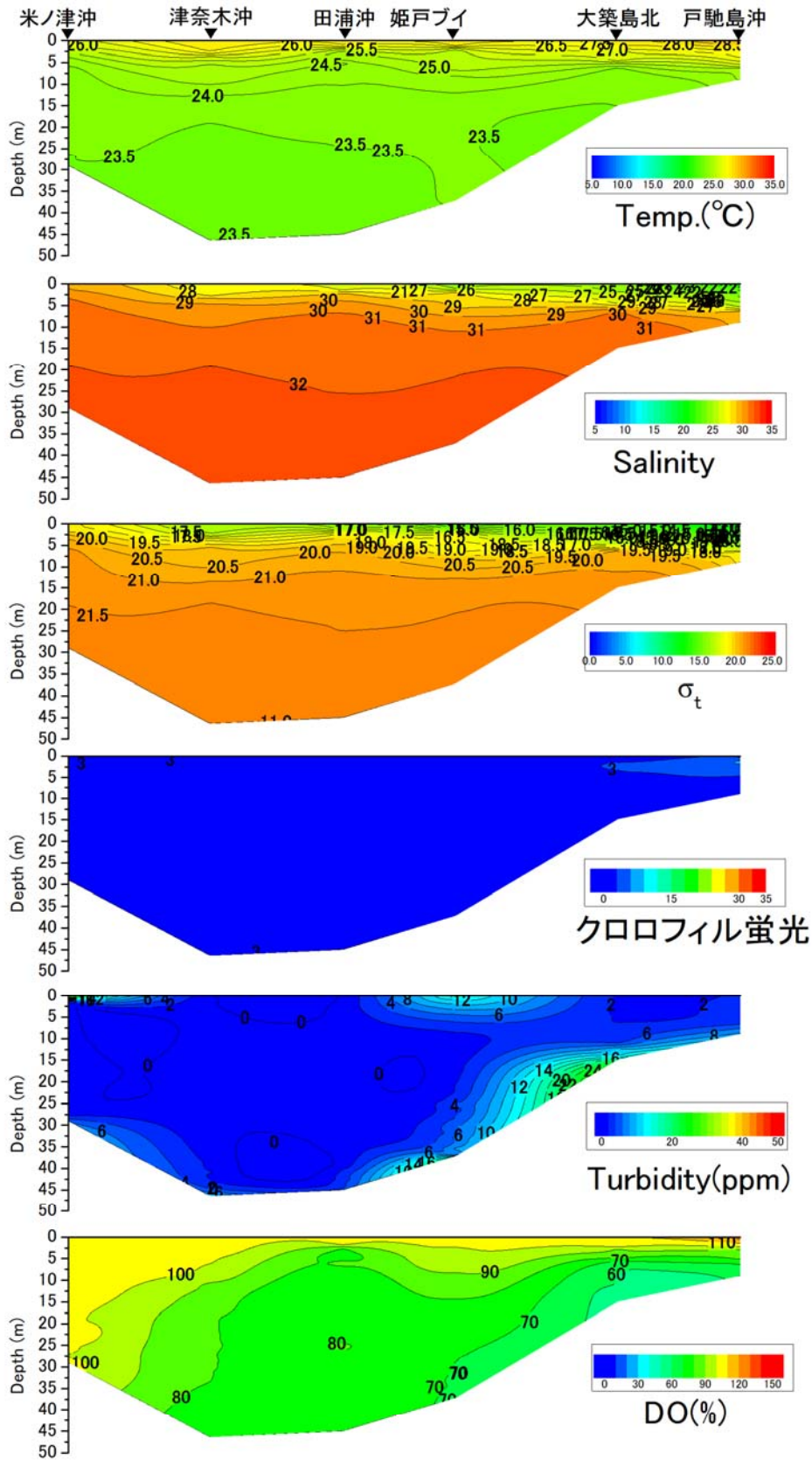
戸馳島沖から米ノ津沖の水温(°C)、塩分、密度( \sigma_t )、クロロフィル蛍光強度、濁度、溶存酸素飽和度(DO%)の鉛直面図(東町漁業協同組合の調査による) (2018年7月17日)
