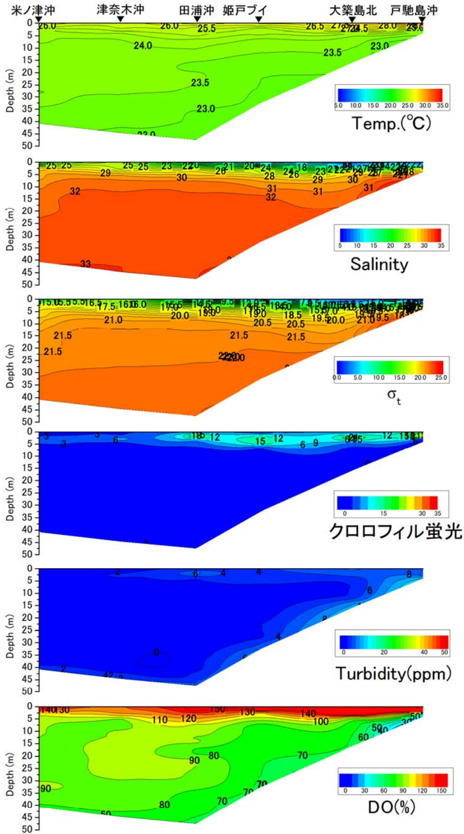
戸馳島沖から米ノ津沖の水温(°C)、塩分、密度( \sigma_t )、クロロフィル蛍光強度、濁度、溶存酸素飽和度(DO%)の鉛直面図(鹿児島県水産技術開発センターの調査による)(2018年7月11日)
