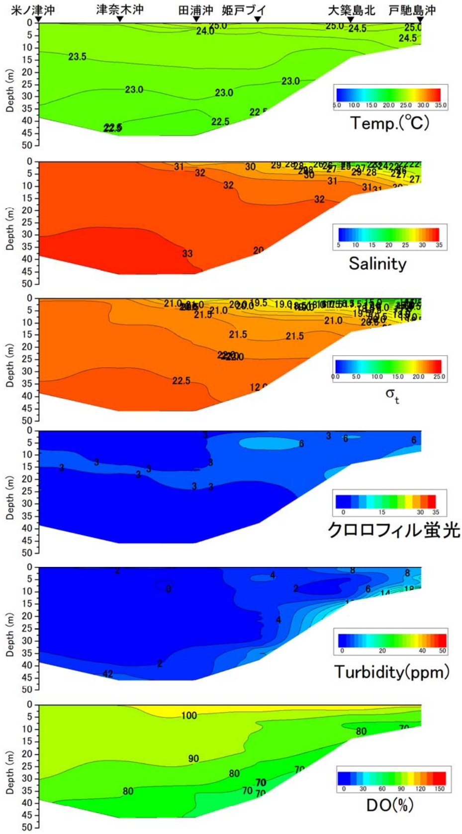
戸馳島沖から米ノ津沖の水温(°C)、塩分、密度( \sigma_t )、クロロフィル蛍光強度、濁度、溶存酸素飽和度(DO%)の鉛直面図(熊本県水産研究センターの調査による)(2018年7月4日)
