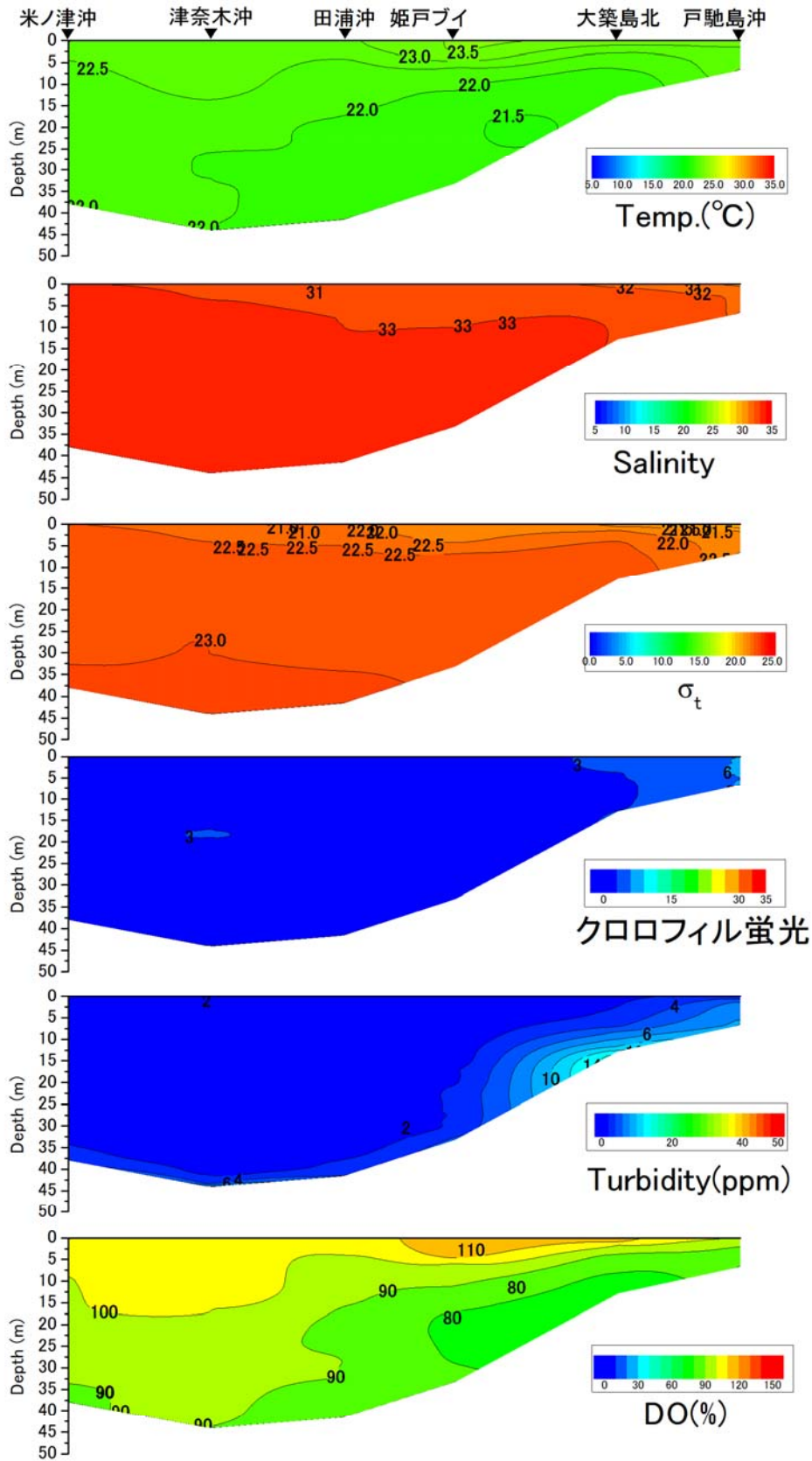
戸馳島沖から米ノ津沖の水温(°C)、塩分、密度( \sigma_t )、クロロフィル蛍光強度、濁度、溶存酸素飽和度(DO%)の鉛直面図(鹿児島県水産技術開発センターの調査による)(2018年6月19日)
