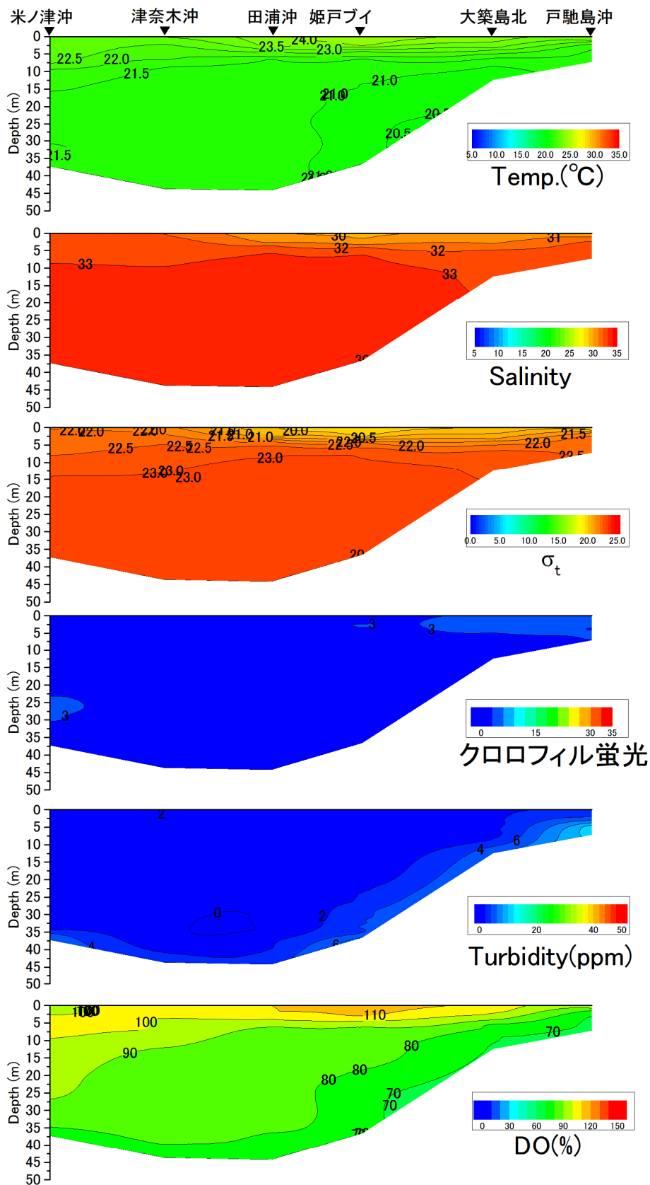
戸馳島沖から米ノ津沖の水温(°C)、塩分、密度( \sigma_t )、クロロフィル蛍光強度、濁度、溶存酸素飽和度(DO%)の鉛直面図(熊本県水産研究センターの調査による)(2018年6月11日)
