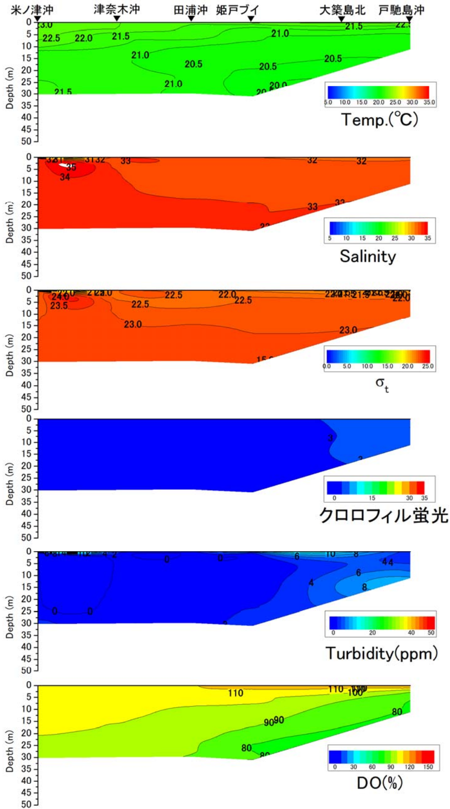
戸馳島沖から米ノ津沖の水温(°C)、塩分、密度( \sigma_t )、クロロフィル蛍光強度、濁度、溶存酸素飽和度(DO%)の鉛直面図(東町漁業協同組合の調査による) (2018年6月5日)
