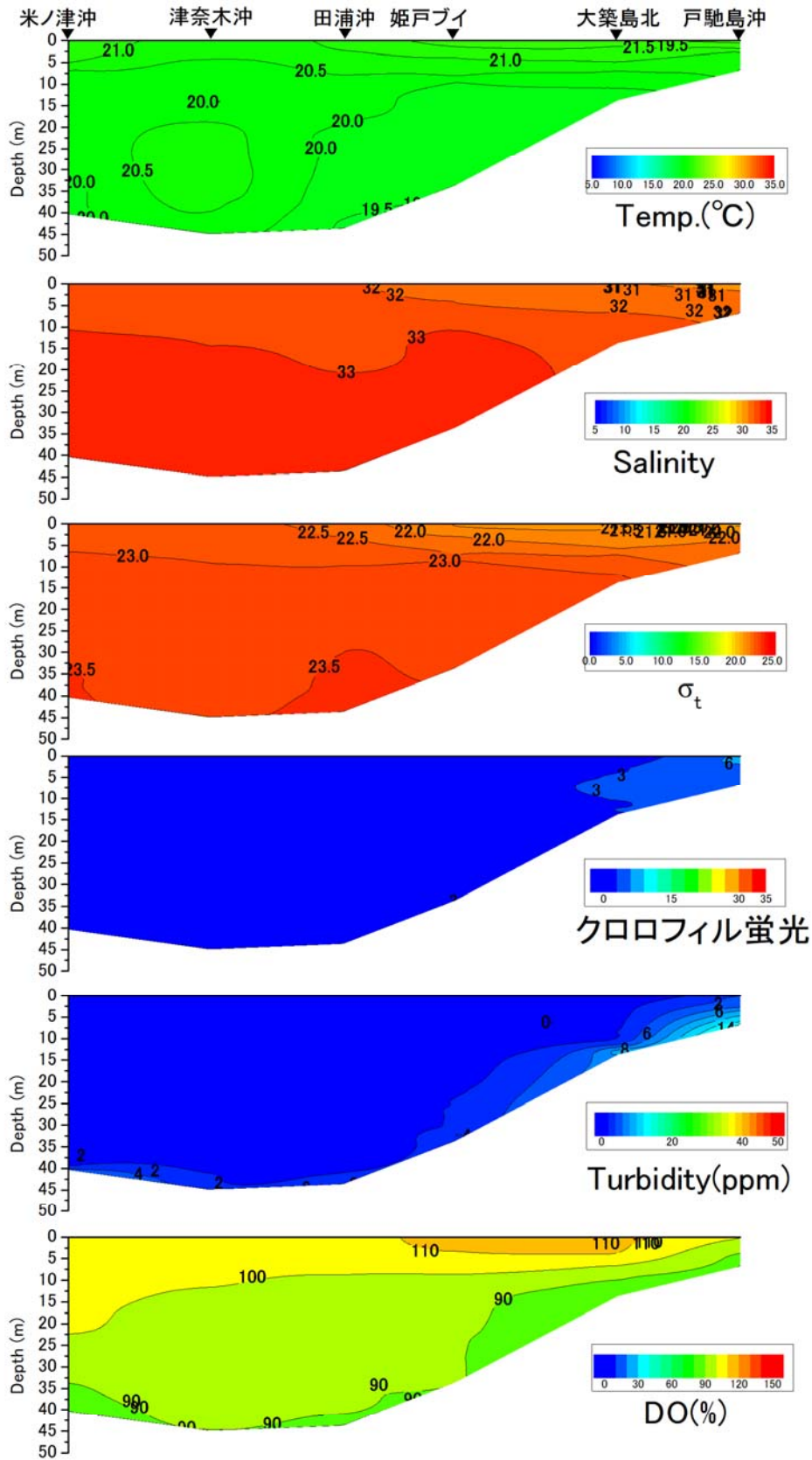
戸馳島沖から米ノ津沖の水温(°C)、塩分、密度( \sigma_t )、クロロフィル蛍光強度、濁度、溶存酸素飽和度(DO%)の鉛直面図(鹿児島県水産技術開発センターの調査による)(2018年5月29日)
