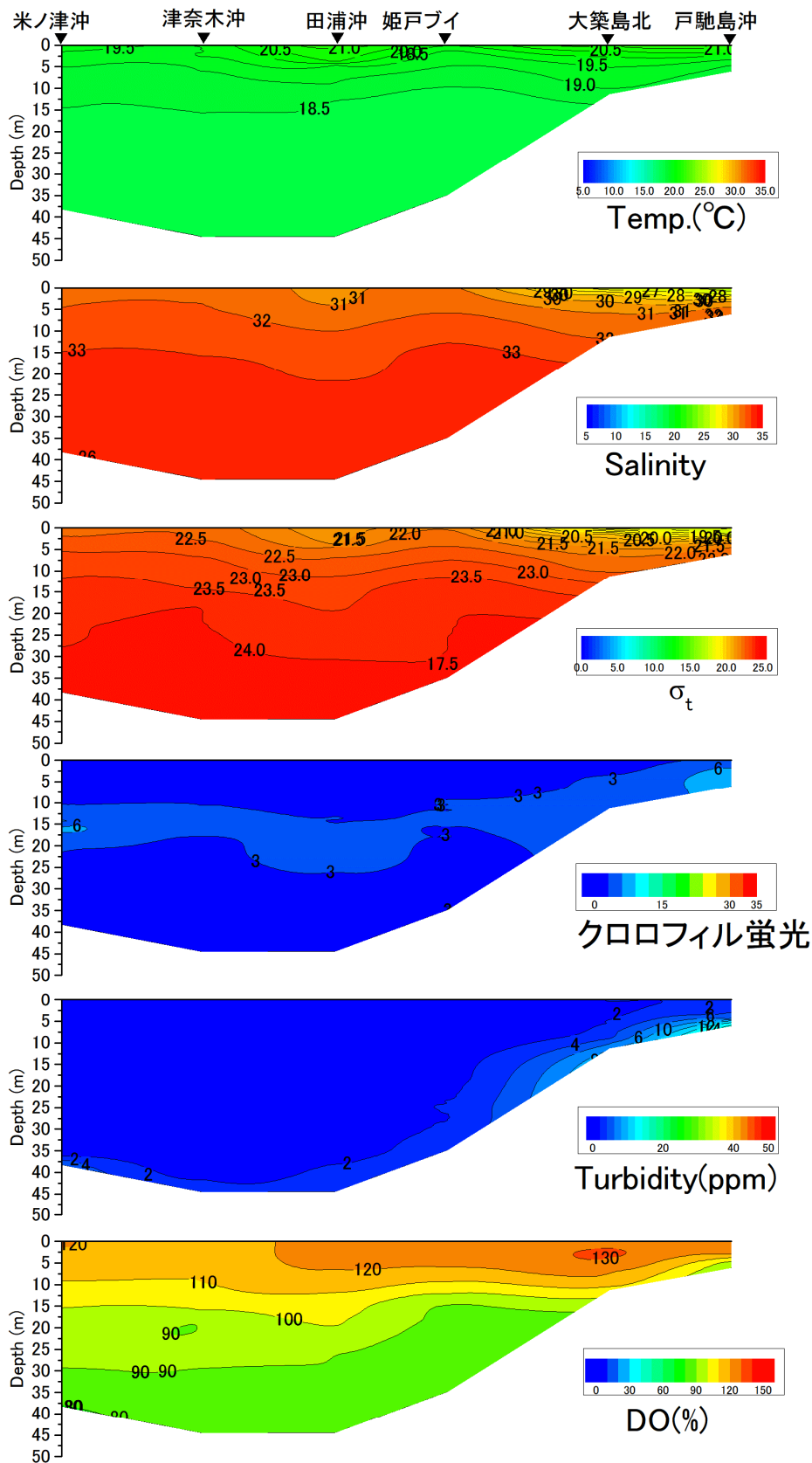
戸馳島沖から米ノ津沖の水温(°C)、塩分、密度( \sigma_t )、クロロフィル蛍光強度、濁度、溶存酸素飽和度(DO%)の鉛直面図(熊本県水産研究センターの調査による)(2018年5月14日)
