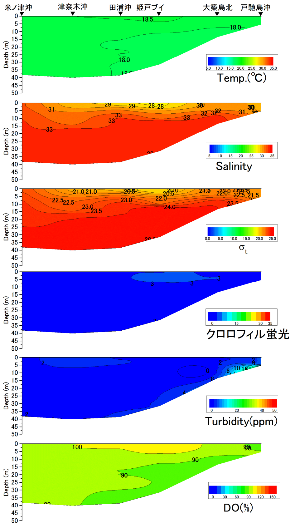
戸馳島沖から米ノ津沖の水温(°C)、塩分、密度( \sigma_t )、クロロフィル蛍光強度、濁度、溶存酸素飽和度(DO%)の鉛直面図(鹿児島県水産技術開発センターの調査による)(2018年5月9日)
