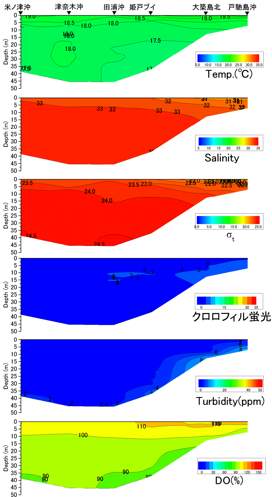
戸馳島沖から米ノ津沖の水温(°C)、塩分、密度( \sigma_t )、クロロフィル蛍光強度、濁度、溶存酸素飽和度(DO%)の鉛直面図(熊本県水産研究センターの調査による)(2018年5月1日)
