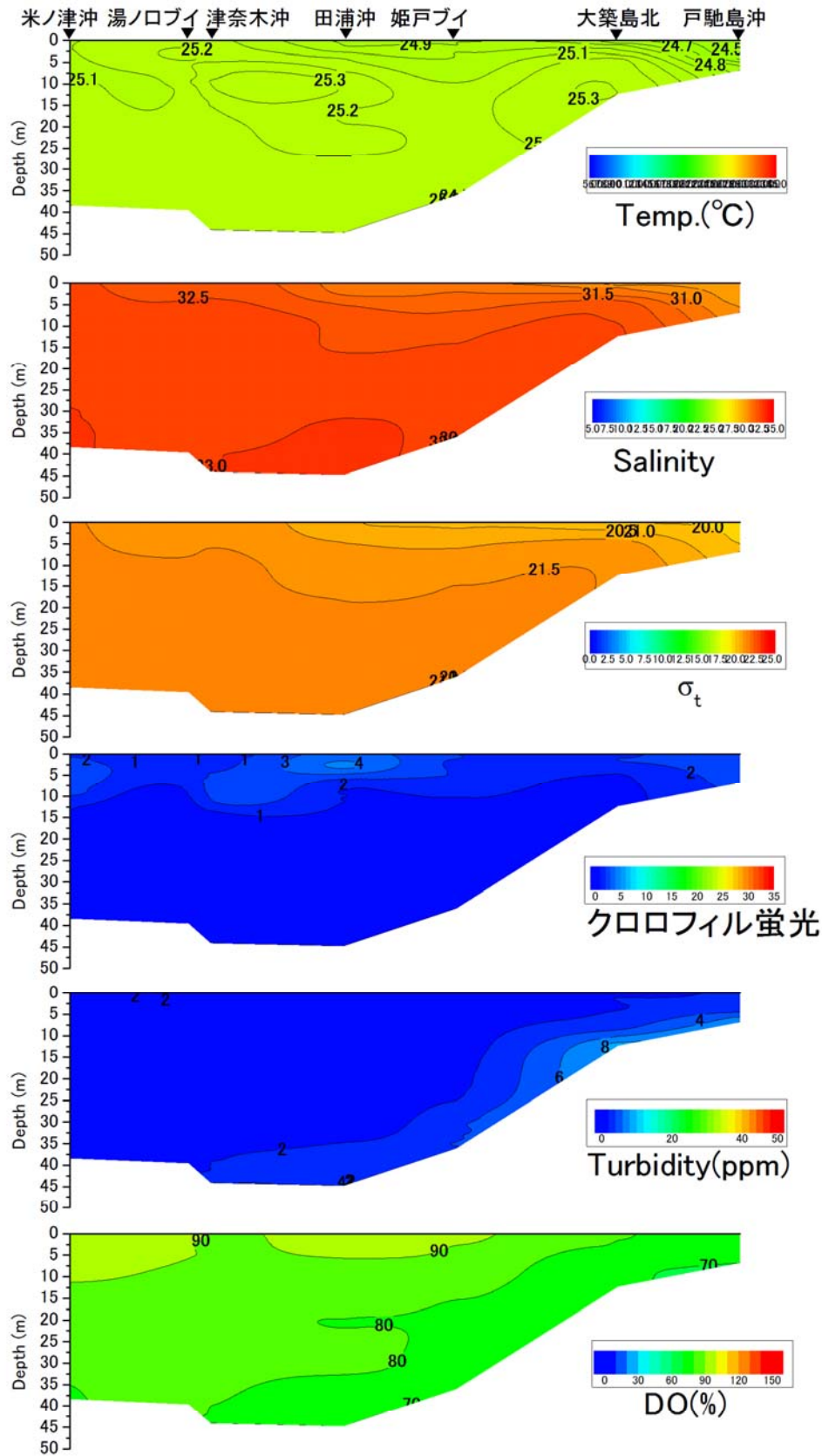
戸馳島沖から米ノ津沖の水温(°C)、塩分、密度( \sigma_t )、クロロフィル蛍光強度、濁度、溶存酸素飽和度(DO%)の鉛直面図(熊本県水産研究センターの調査による)(2017年9月26日)
