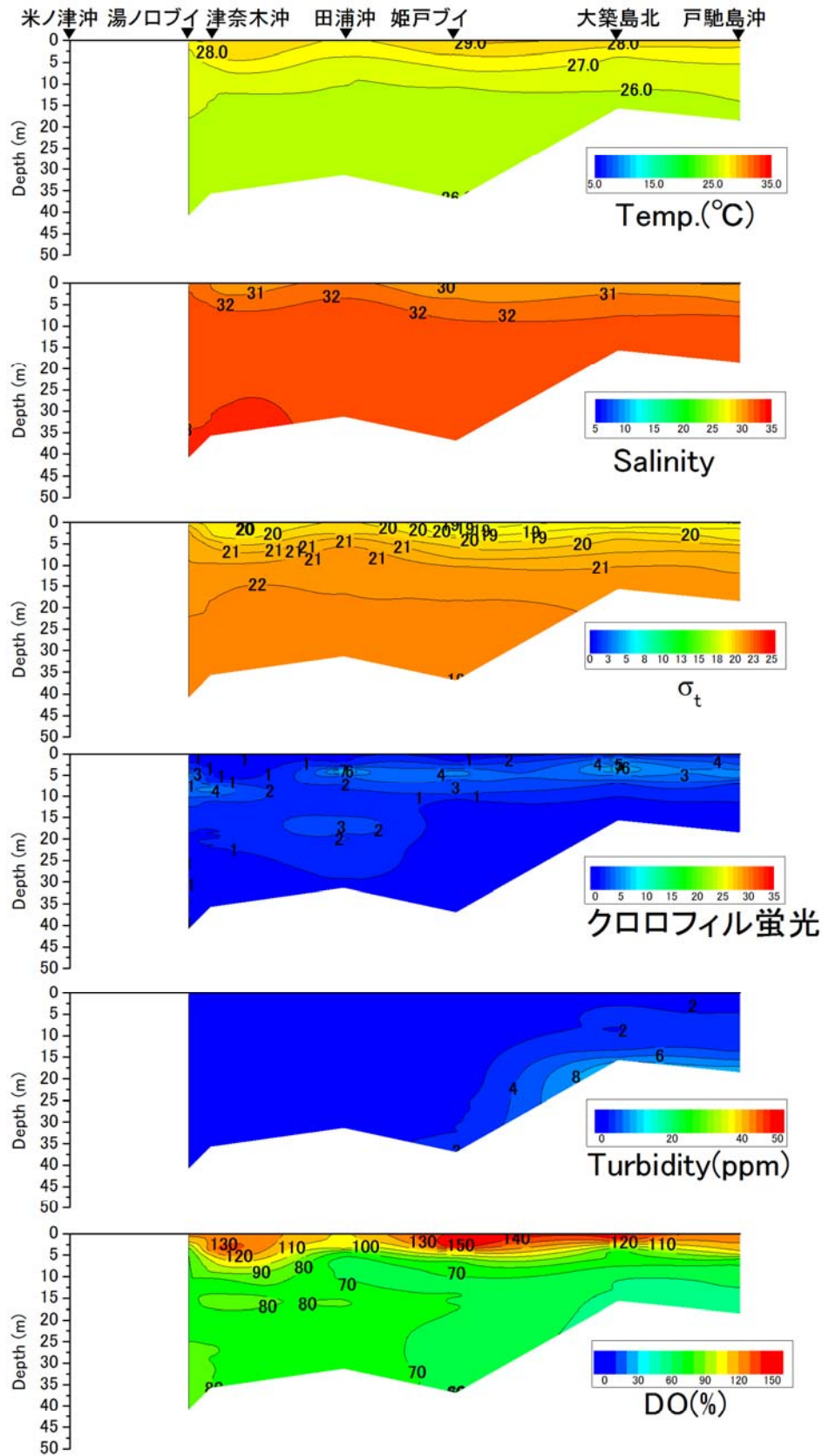
戸馳島沖から津奈木沖の水温(°C)、塩分、密度( \sigma_t )、クロロフィル蛍光強度、濁度、溶存酸素飽和度(DO%)の鉛直面図(東町漁業協同組合の調査による) (2017年8月29日)
