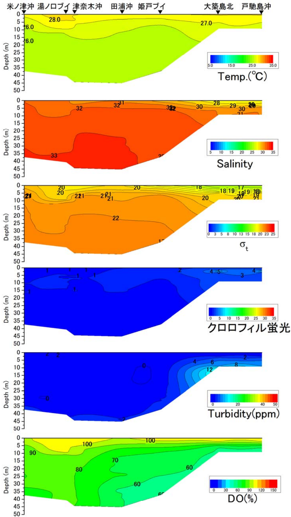
戸馳島沖から津奈木沖の水温(°C)、塩分、密度( \sigma_t )、クロロフィル蛍光強度、濁度、溶存酸素飽和度(DO%)の鉛直面図(熊本県水産研究センターの調査による)(2017年8月22日)
