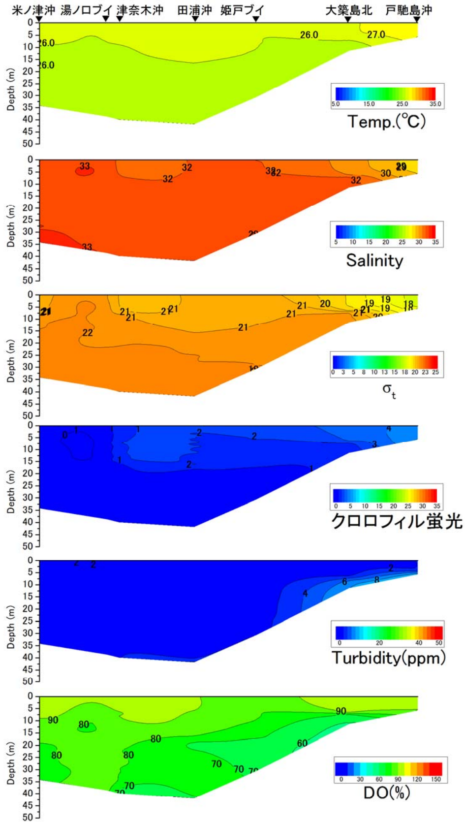
戸馳島沖から津奈木沖の水温(°C)、塩分、密度( \sigma_t )、クロロフィル蛍光強度、濁度、溶存酸素飽和度(DO%)の鉛直面図(鹿児島県水産技術開発センターの調査による)(2017年8月15日)
