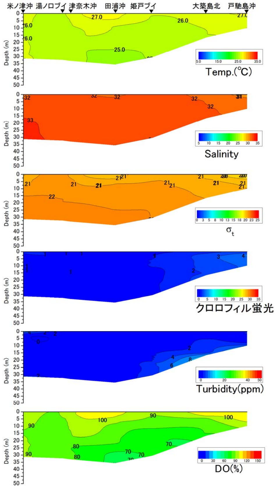
戸馳島沖から津奈木沖の水温(°C)、塩分、密度( \sigma_t )、クロロフィル蛍光強度、濁度、溶存酸素飽和度(DO%)の鉛直面図(東町漁業協同組合の調査による) (2017年8月10日)
