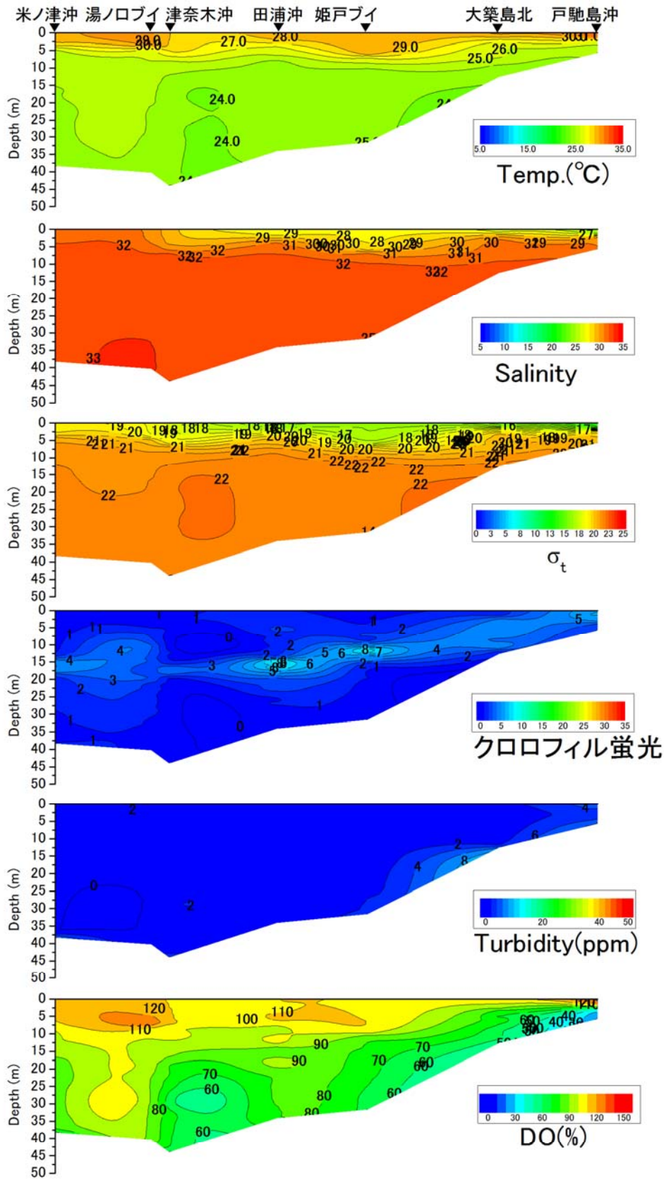
戸馳島沖から津奈木沖の水温(°C)、塩分、密度( \sigma_t )、クロロフィル蛍光強度、濁度、溶存酸素飽和度(DO%)の鉛直面図(鹿児島県水産技術開発センターの調査による)(2017年8月2日)
