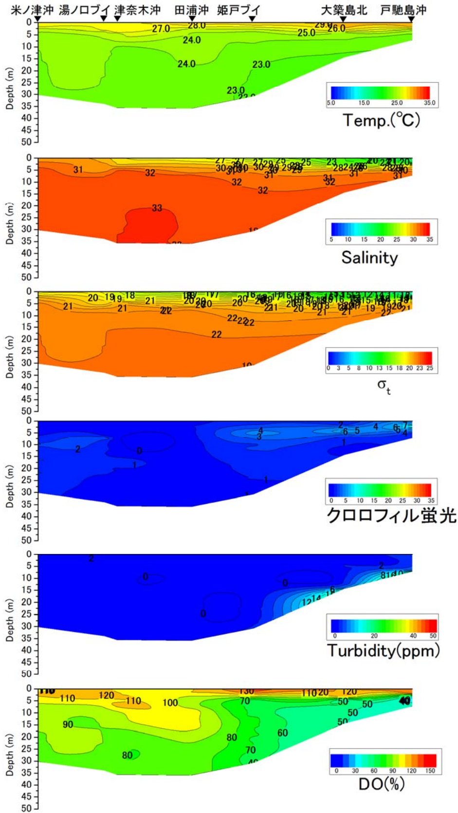
戸馳島沖から津奈木沖の水温(°C)、塩分、密度( \sigma_t )、クロロフィル蛍光強度、濁度、溶存酸素飽和度(DO%)の鉛直面図(東町漁業協同組合の調査による) (2017年7月18日)
