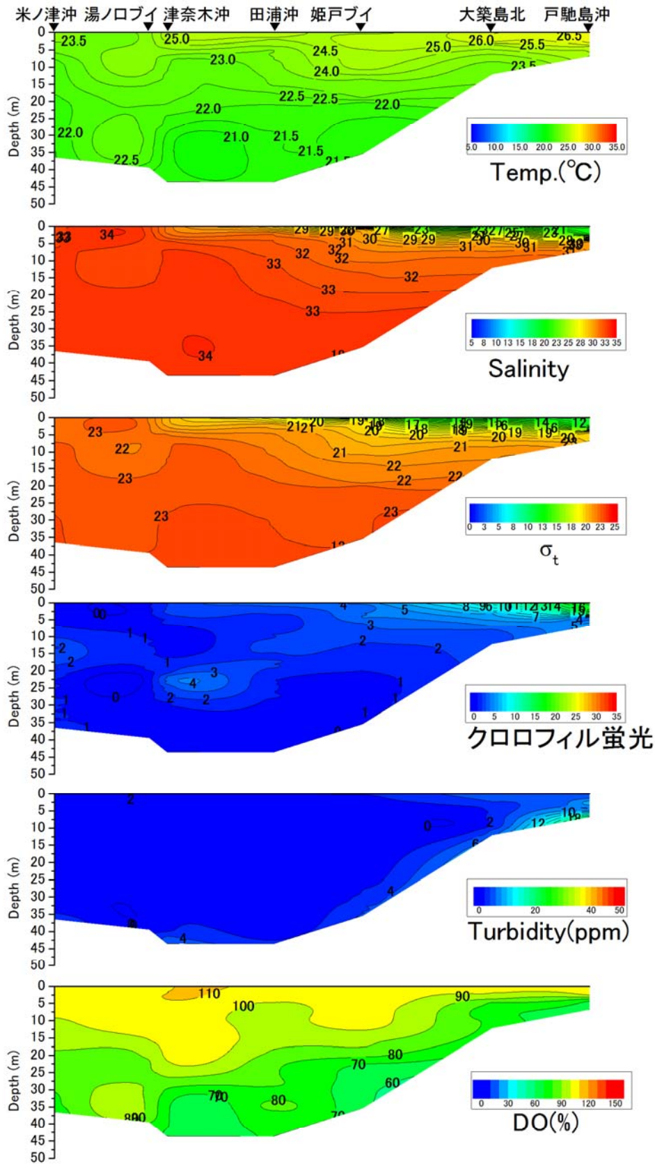
戸馳島沖から津奈木沖の水温(°C)、塩分、密度( \sigma_t )、クロロフィル蛍光強度、濁度、溶存酸素飽和度(DO%)の鉛直面図(熊本県水産研究センターの調査による)(2017年7月6日)
