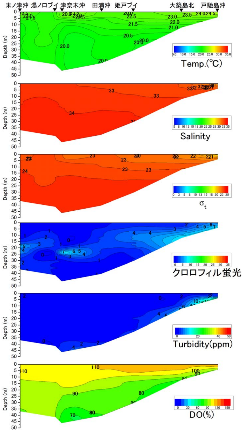
戸馳島沖から米ノ津沖の水温(°C)、塩分、密度( \sigma_t )、クロロフィル蛍光強度、濁度、溶存酸素飽和度(DO%)の鉛直面図(鹿児島県水産技術開発センターの調査による)(2017年6月20日)
