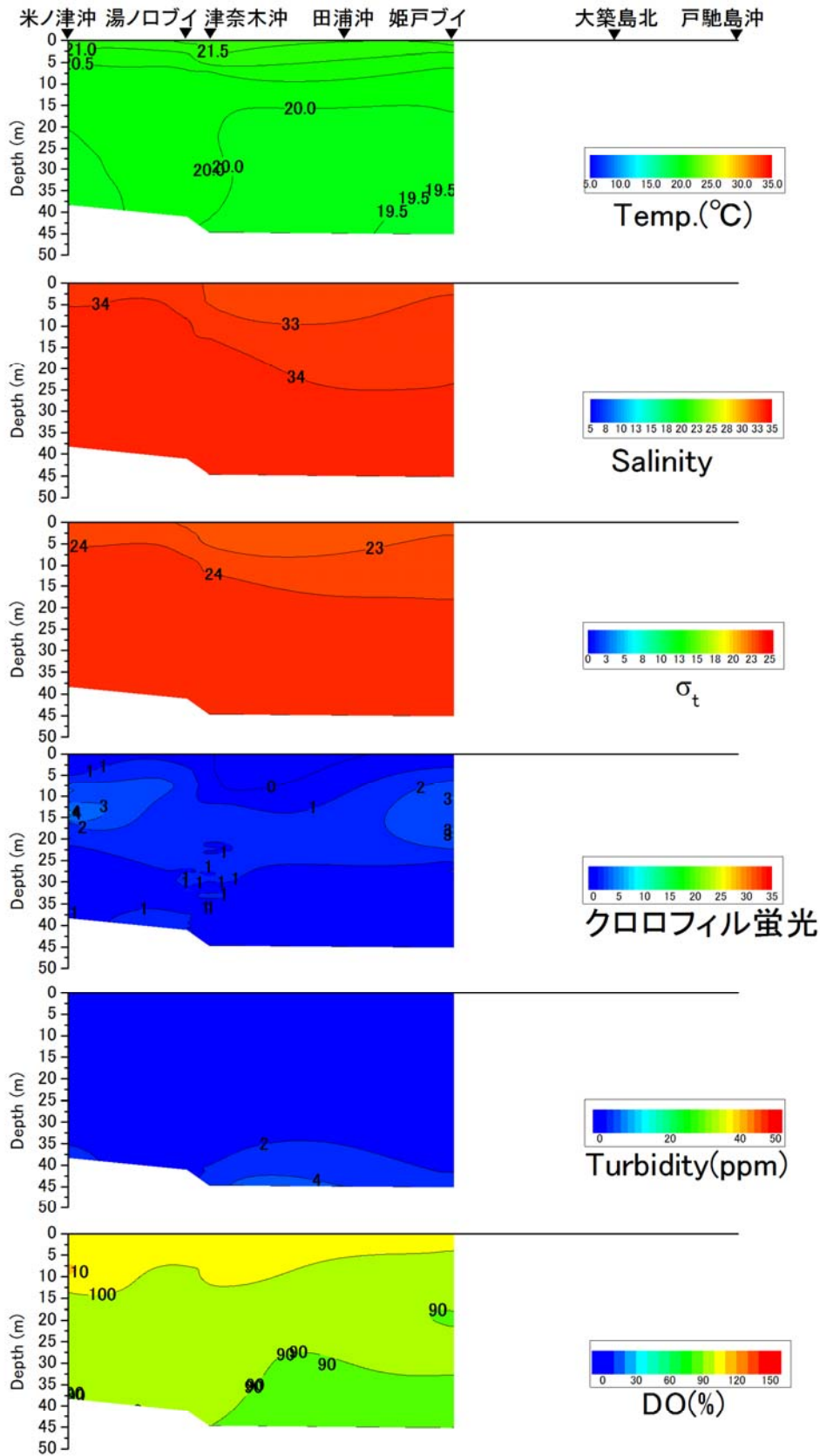
戸馳島沖から津奈木沖の水温(°C)、塩分、密度( \sigma_t )、クロロフィル蛍光強度、濁度、溶存酸素飽和度(DO%)の鉛直面図(熊本県水産研究センターの調査による)(2017年6月12日)
