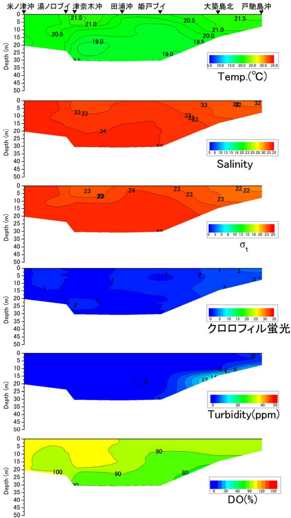
戸馳島沖から津奈木沖の水温(°C)、塩分、密度( \sigma_t )、クロロフィル蛍光強度、濁度、溶存酸素飽和度(DO%)の鉛直面図(東町漁業協同組合の調査による) (2017年6月7日)
