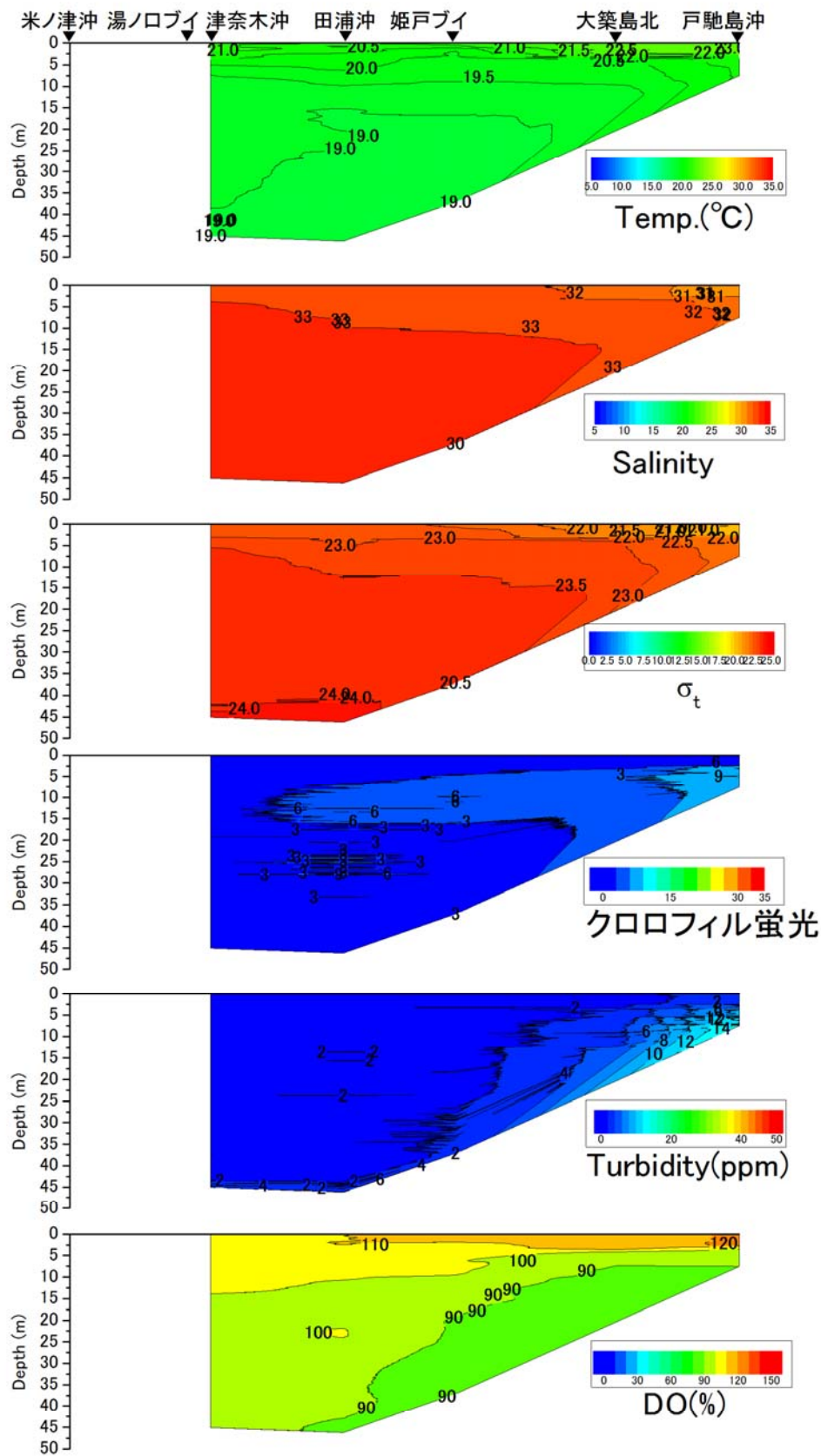
戸馳島沖から津奈木沖の水温(°C)、塩分、密度( \sigma_t )、クロロフィル蛍光強度、濁度、溶存酸素飽和度(DO%)の鉛直面図(熊本県水産研究センターの調査による)(2017年5月30日)
