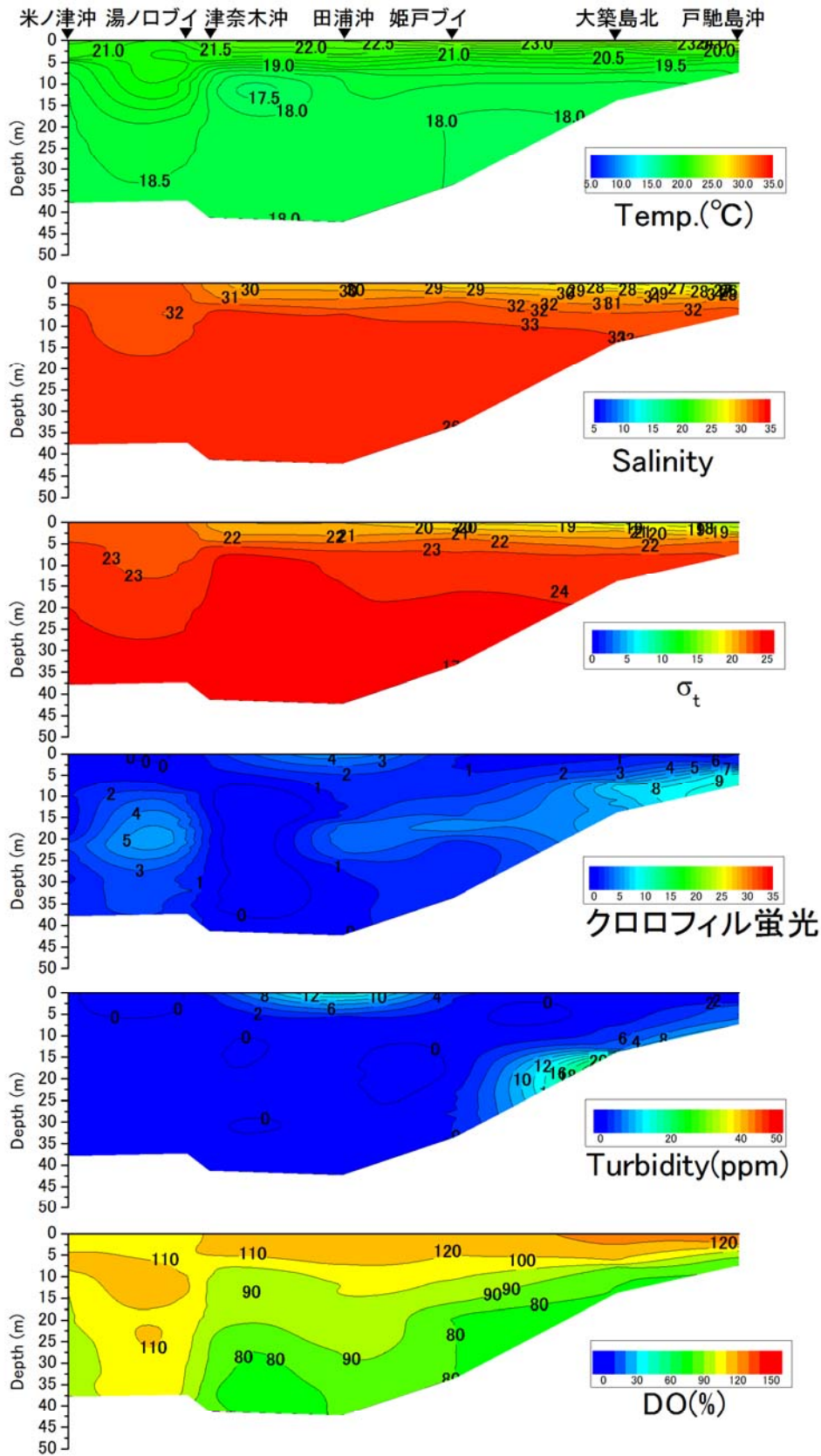
戸馳島沖から米ノ津沖の水温(°C)、塩分、密度( \sigma_t )、クロロフィル蛍光強度、濁度、溶存酸素飽和度(DO%)の鉛直面図(鹿児島県水産技術開発センターの調査による)(2017年5月23日)
