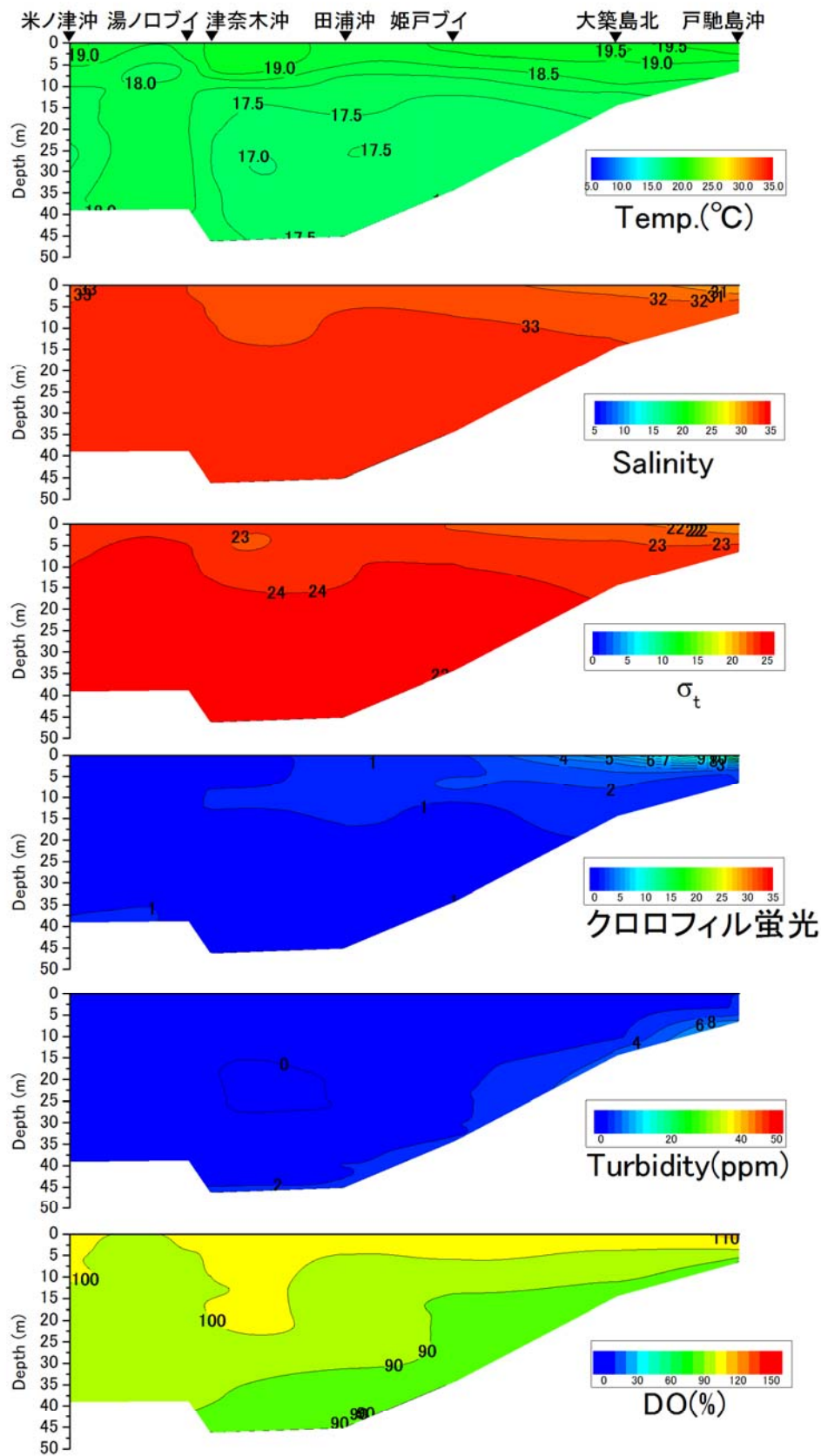
戸馳島沖から米ノ津沖の水温(°C)、塩分、密度( \sigma_t )、クロロフィル蛍光強度、濁度、溶存酸素飽和度(DO%)の鉛直面図(熊本県水産研究センターの調査による)(2017年5月9日)
